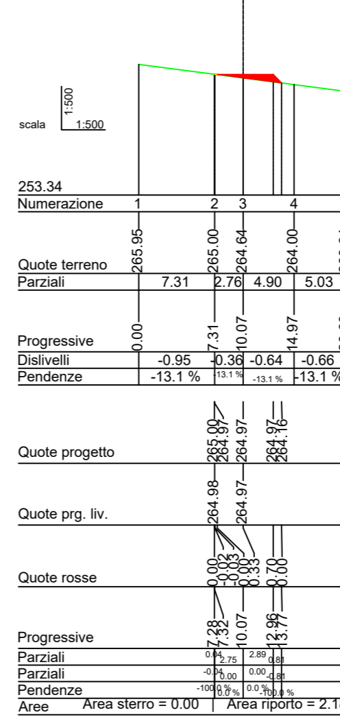
Sez_34 Prog.=675.752
