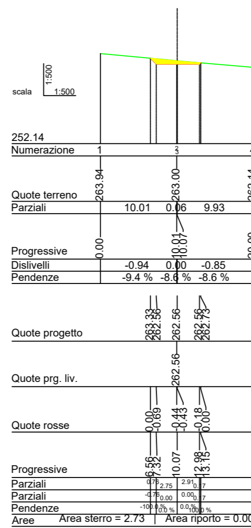
Sez_31 Prog.=615.752
