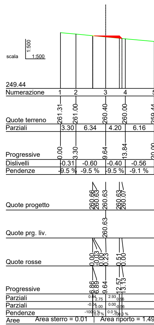
Sez_28 Prog.=555.755
