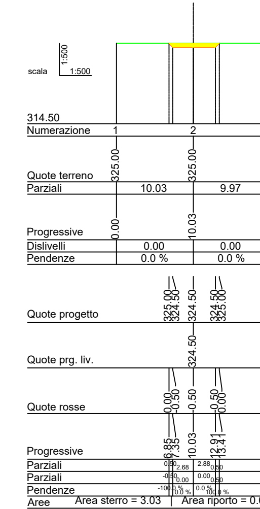
Sez_16 Prog.=293.533
