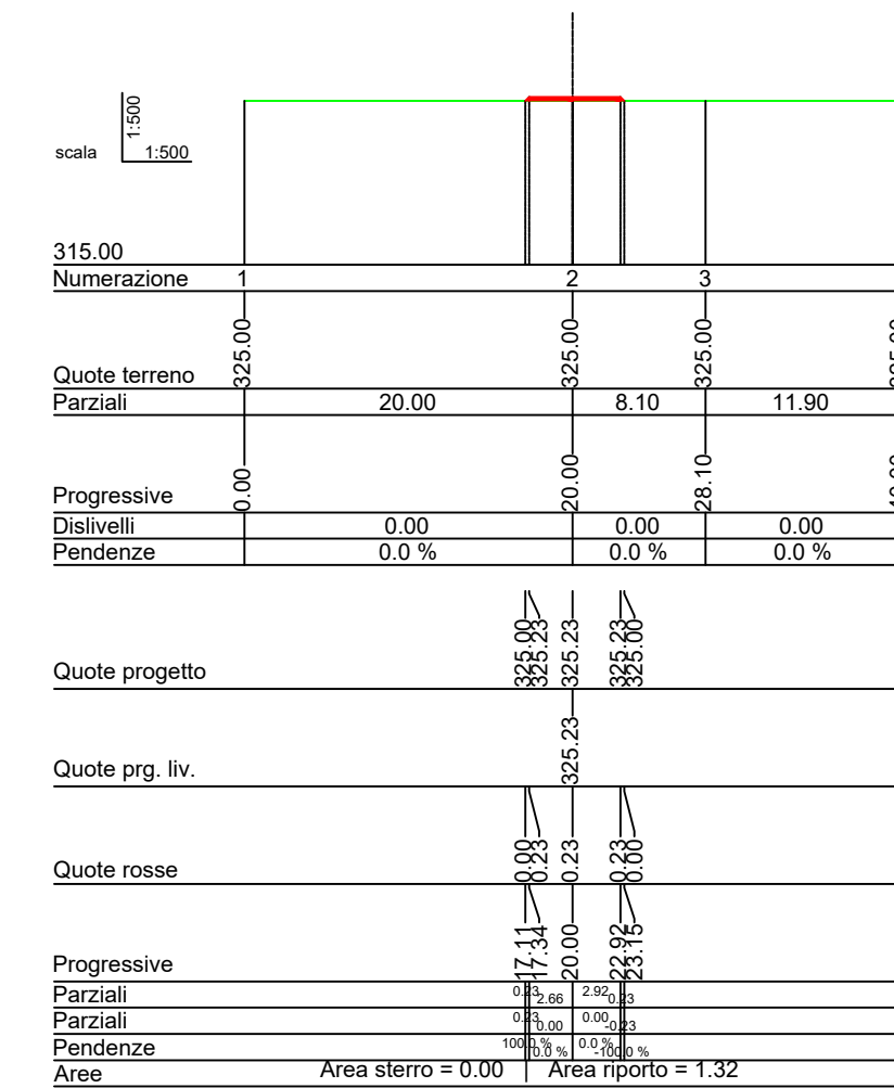
Sez_14 Prog.=253.533
