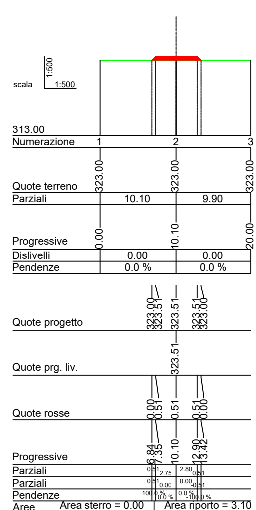
Sez_20 Prog.=373.084
