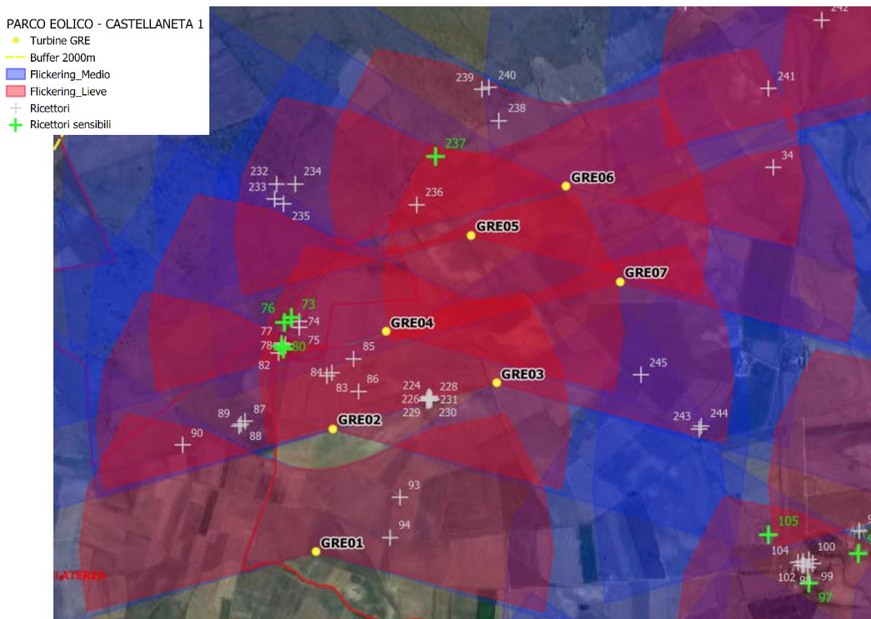
Figura 5-2: Effetto delle turbine GRE01-02-03-04-05-06-07
