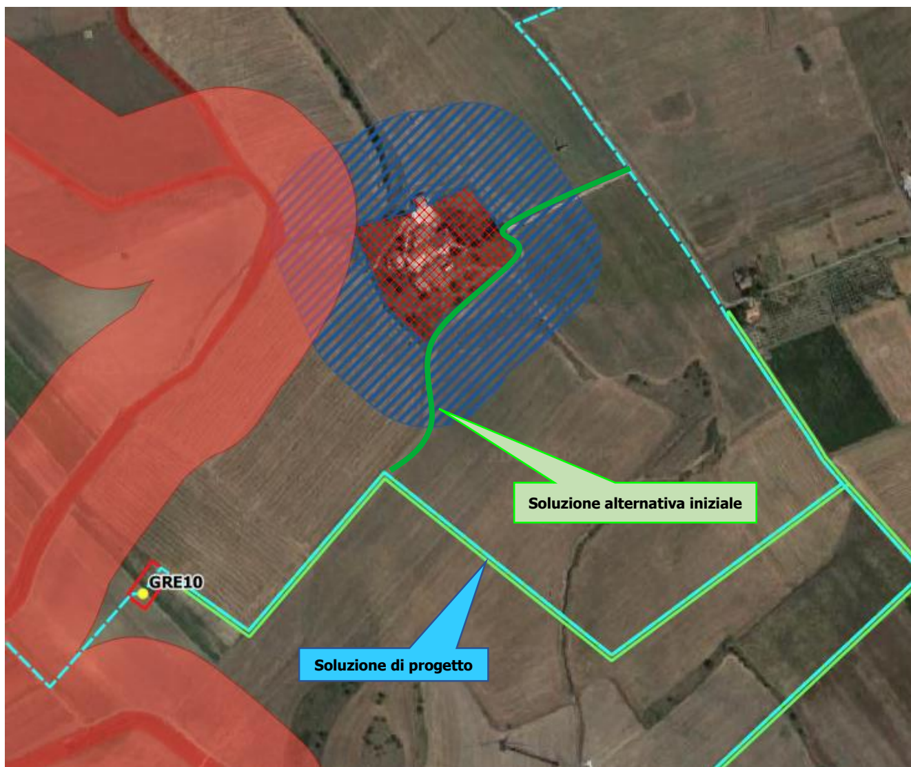
Figura 11-3: Spostamento tracciato cavidotto - Alternativa 2
