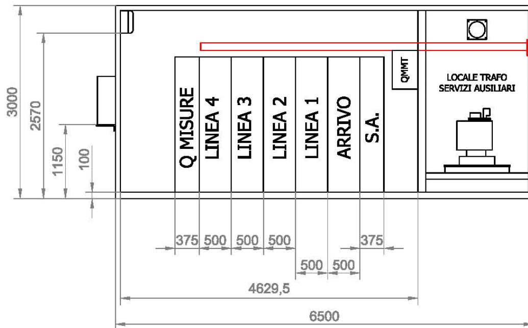
Figura 3-6: Prospetto locale AT in Cabina di Consegna utente
