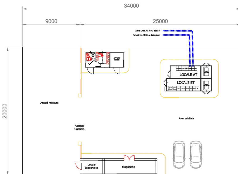
Figura 3-5: Cabina di Consegna utente – schema planimetrico
