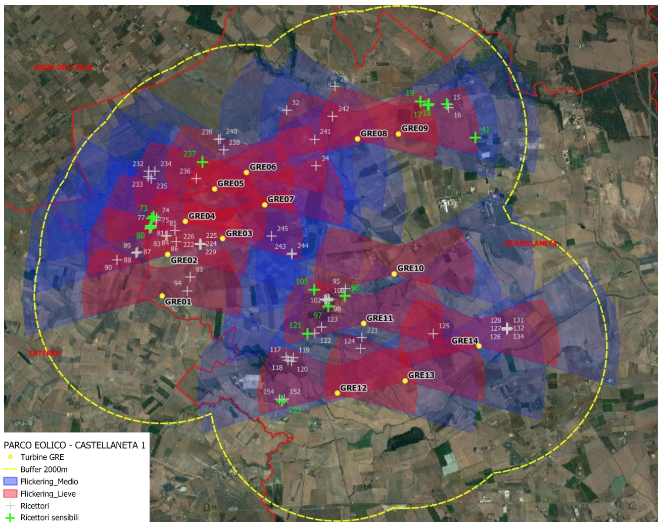
Figura 5-1: Evoluzione dell'ombra nell'area di indagine
