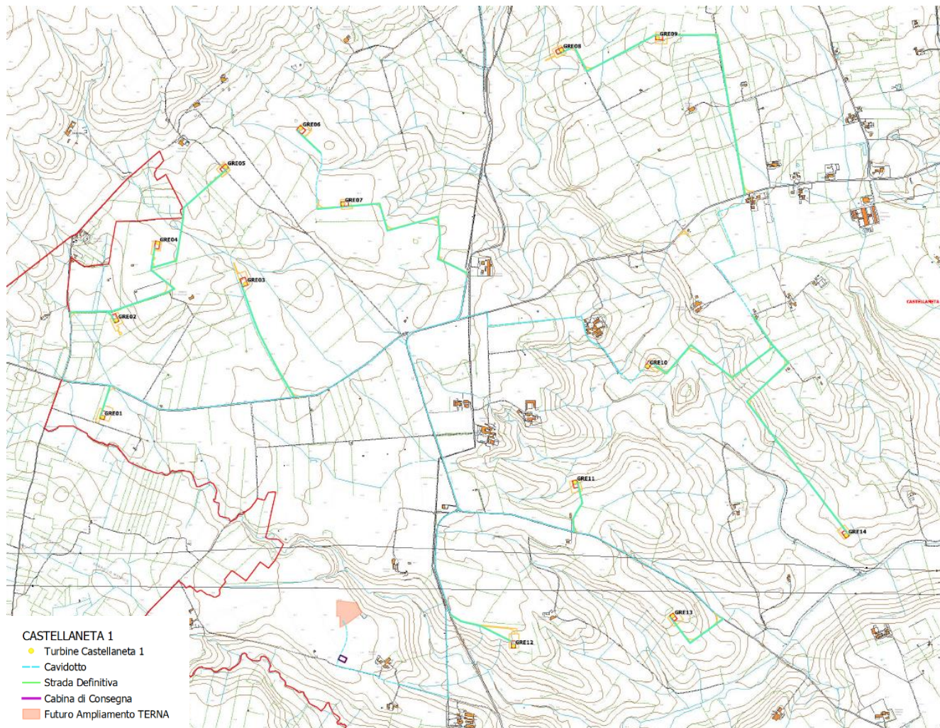
Figura 1-3: Layout del Parco Eolico su base CTR
