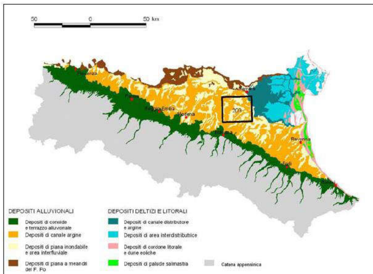
Figura 4 - Inquadramento dei principali ambienti deposizionali del Foglio 203. Tratto dalla “Carta geologica di pianura dell’Emilia-Romagna, in scala 1:250.000”, Regione Emilia-Romagna, 1999.
