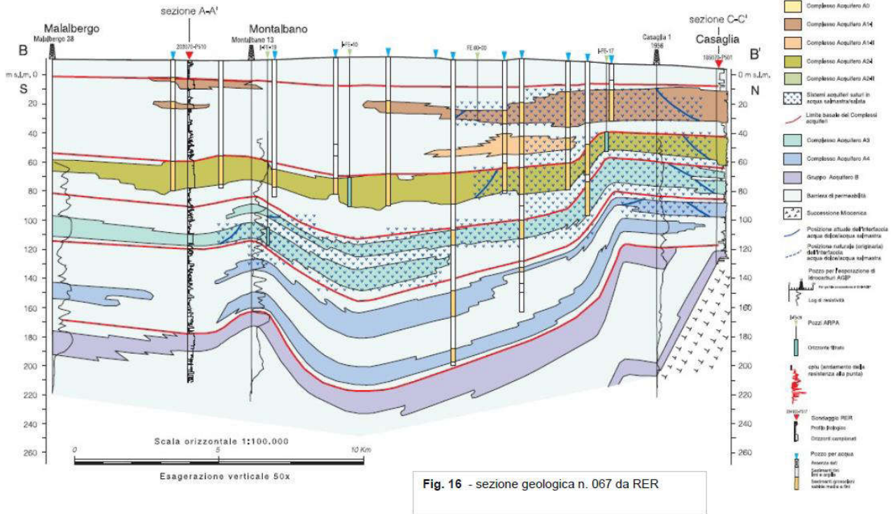
Figura 10 – Sezione geologia n. 067 da RER
