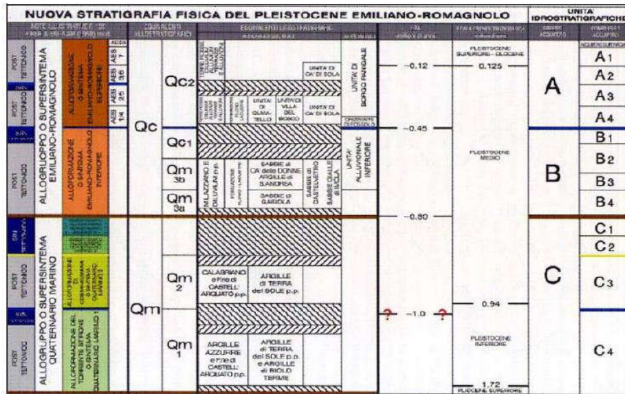
Figura 15 – Schema geologico-stratigrafico del Bacino Pleistocenico della Pianura Emiliano-Romagnola, “Di Dio G. (2001)
