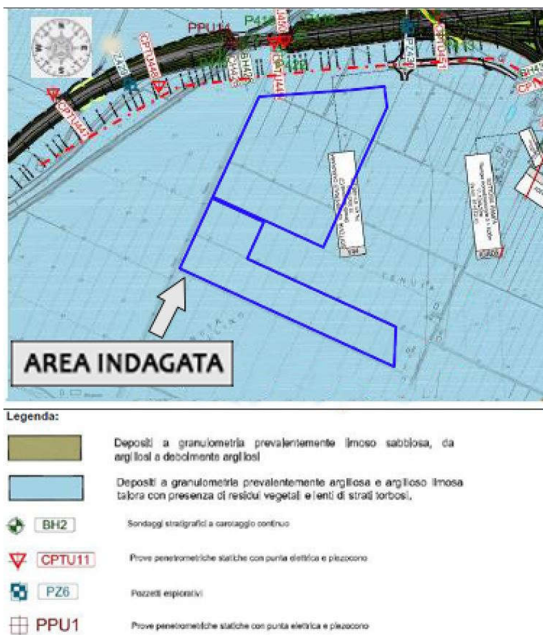
Figura 13 – Stralcio carta geologica, alla scala 1 5.000 rimpicciolita del 90%, dell'area prossima al casello Ferrara sud. Tratto da progetto esecutivo Cispadana. È riportata la traccia (linea tratteggiata) del profilo geologico.
