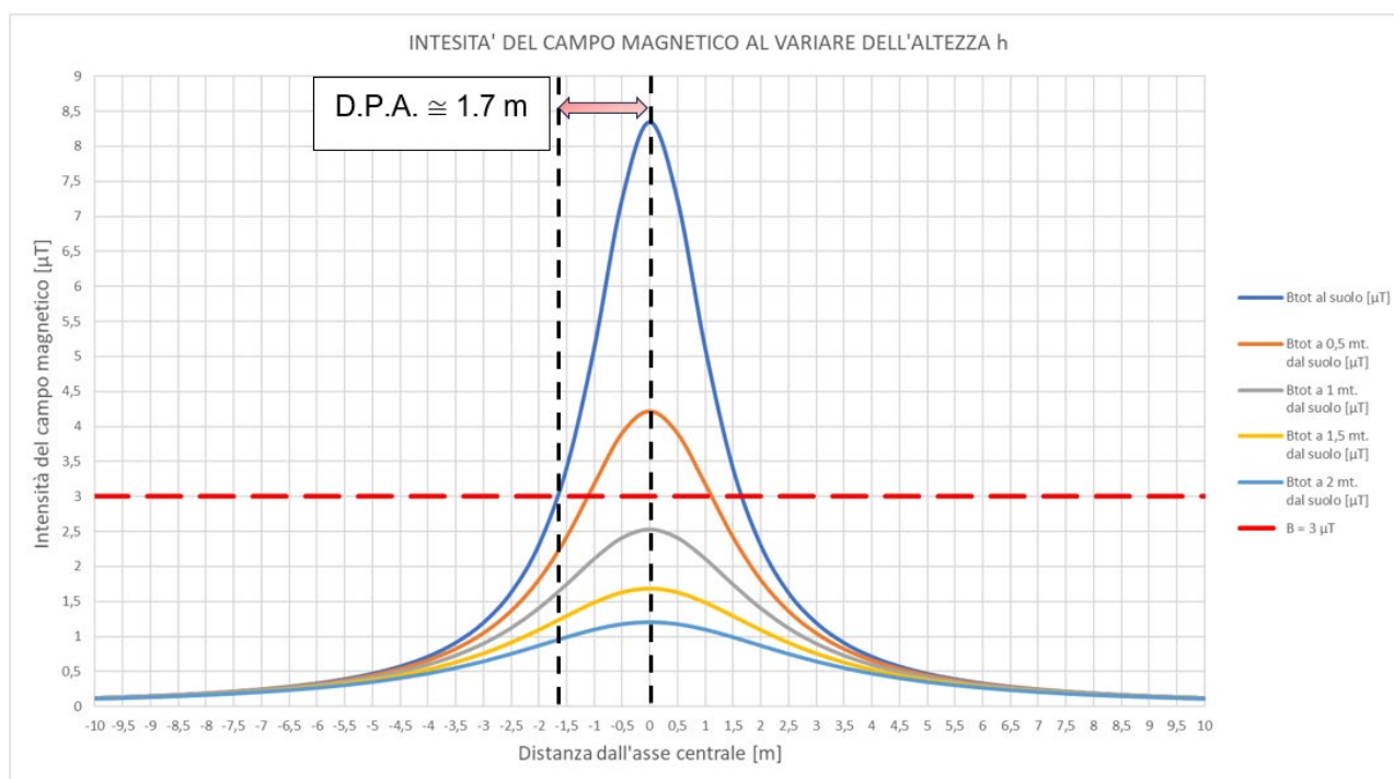
Profilo del Campo di induzione magnetica sulla sezione dei cavi di vettoriamento MT
