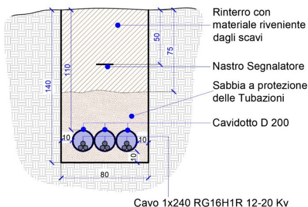
Figura 11 Sezione Tipo Cavidotto Interrato
