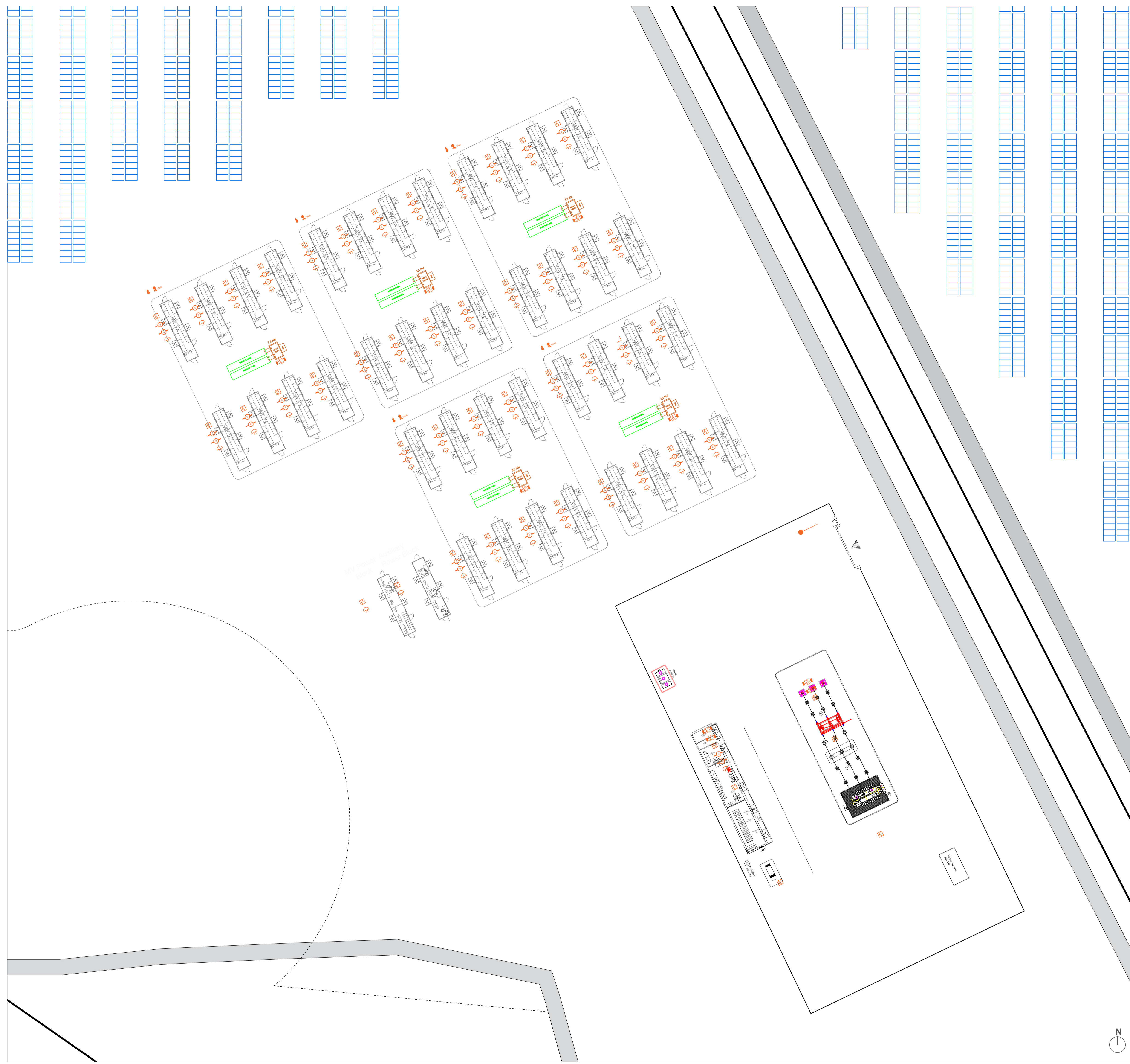
PLANIMETRIA LAYOUT ANTINCENDIO_ Scala 1: 250
