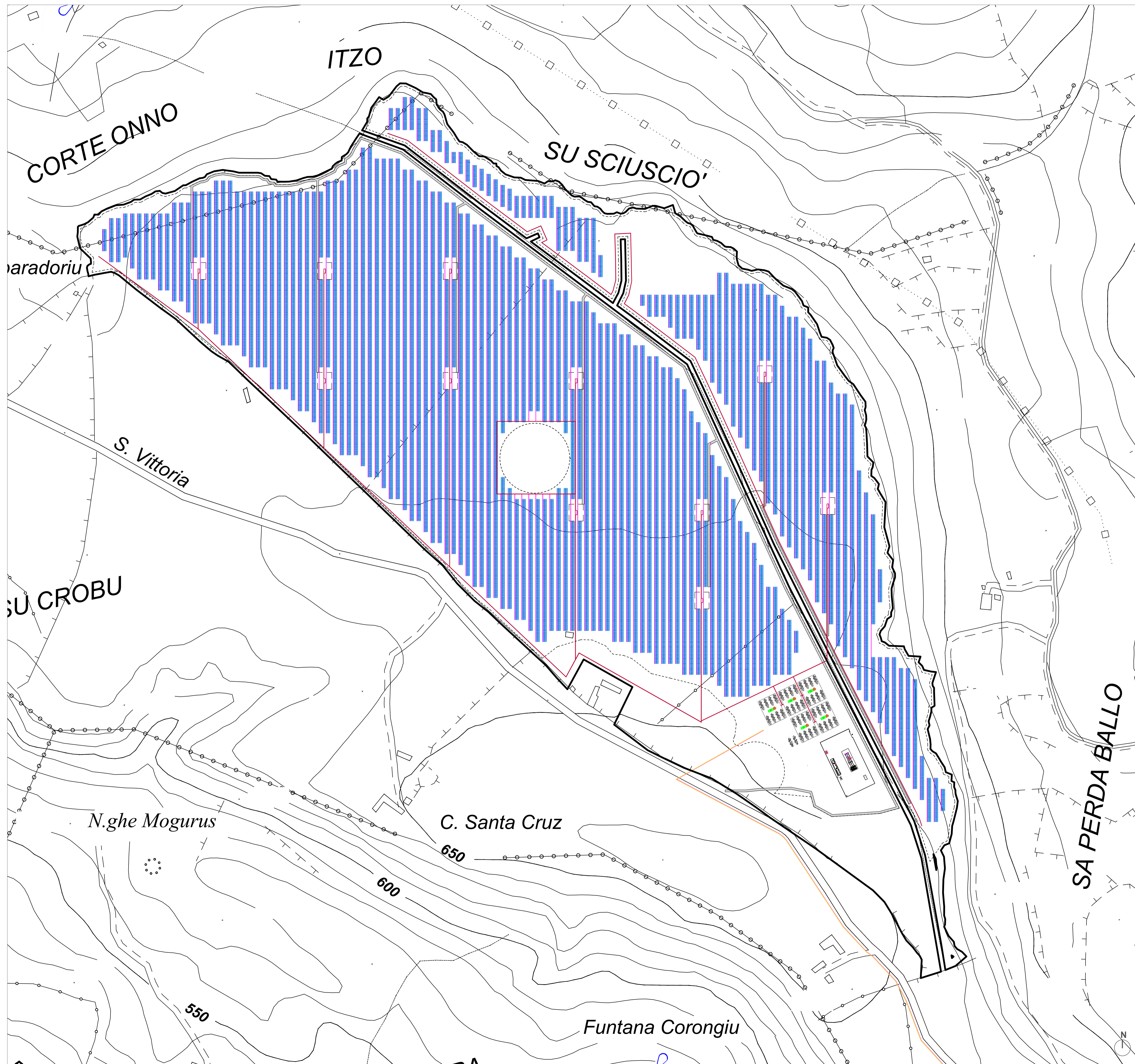
INSERIMENTO LAYOUT_PLANIMETRIA CAVIDOTTI
