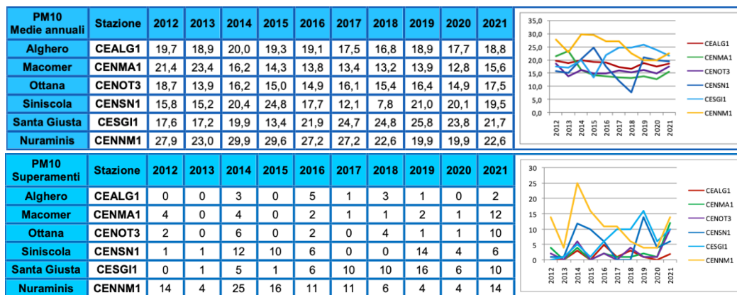
Fig. 18-19: Medie annuali di biossido di PM10 e superamento dei valori ( \mu\text{g}/\text{m}^3 ).
