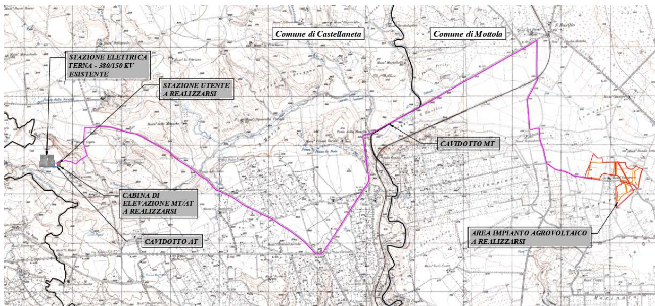
Figura 3 - Percorso cavidotto esterno
