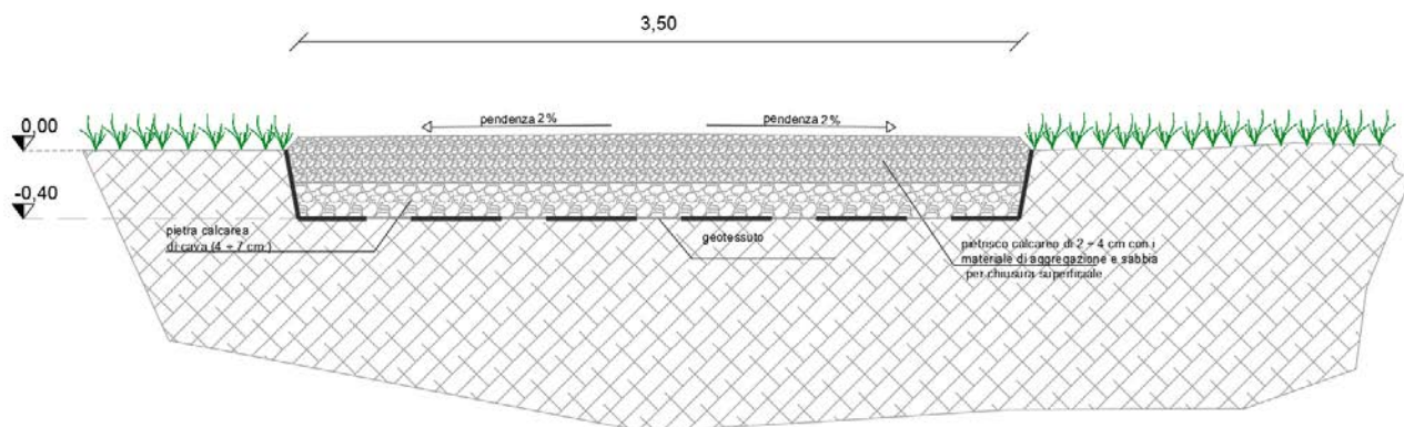
Figura 4 - Sezione tipo viabilità interna
