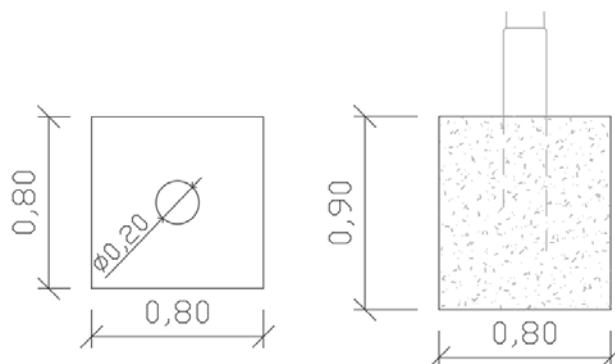
Figura 5 - Particolare costruttivo dello scavo dei pali di illuminazione e videosorveglianza
