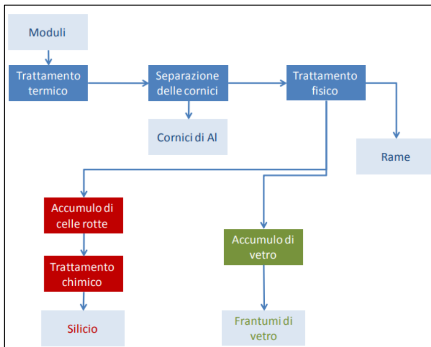
Figura 4: Processo Deutsche Solar
