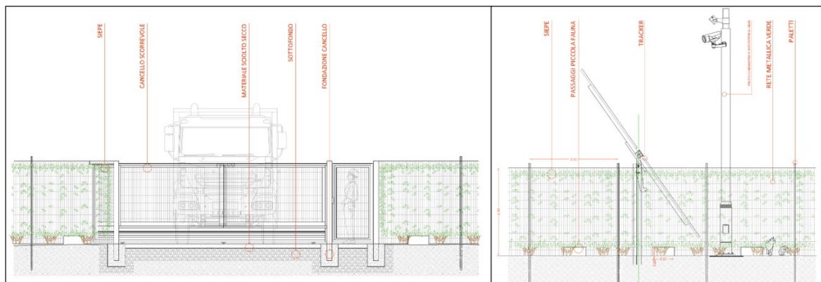
Figura 3: Particolari recinzione, cancelli e impianto di videosorveglianza
