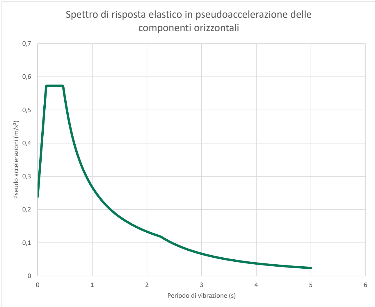
Figura 4: Spettro di risposta elastico in accelerazione delle componenti orizzontali allo stato limite di salvaguardia della vita (SLV)
