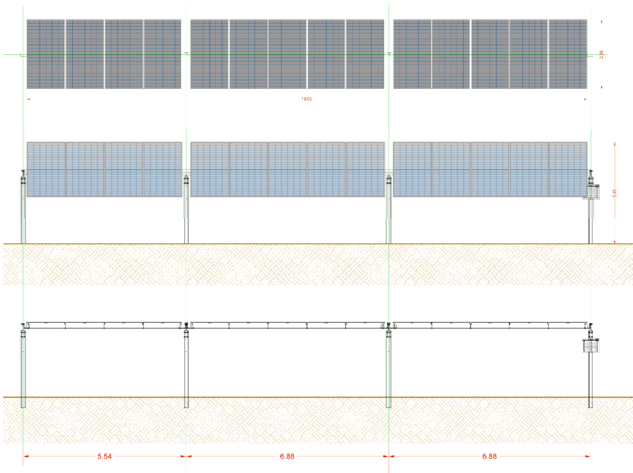
Figura 1: Pianta e prospetti quotati del sistema tracker (inseguitore solare) tipo monoassiale single portrait.
