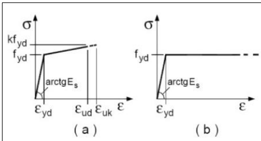
Figura 3 - Diagrammi costitutivi acciaio
