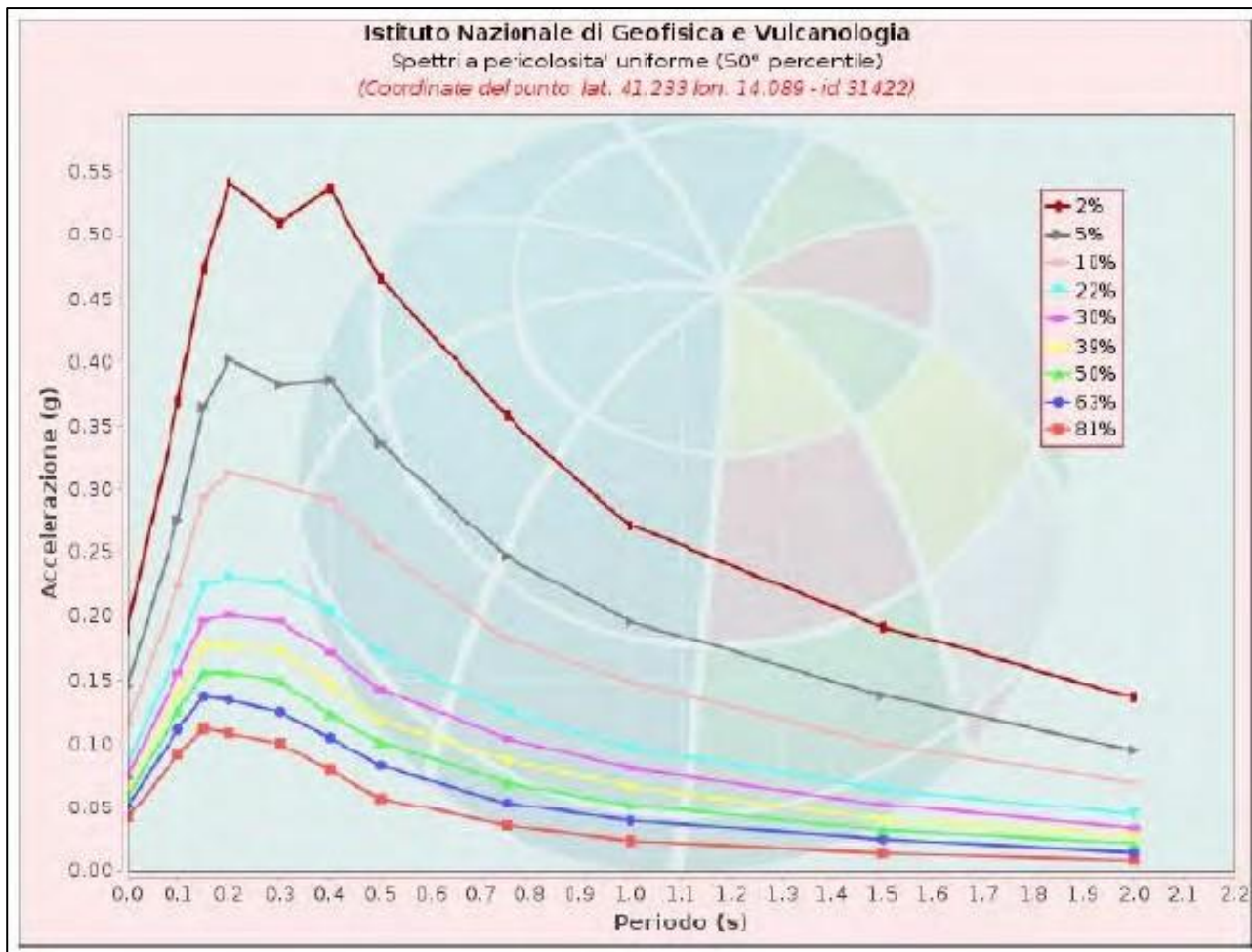
Figura 4 - Spettri di risposta
