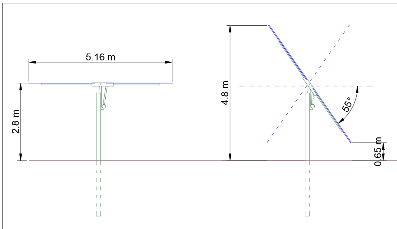
Figura 2 - Schema struttura - sezione
