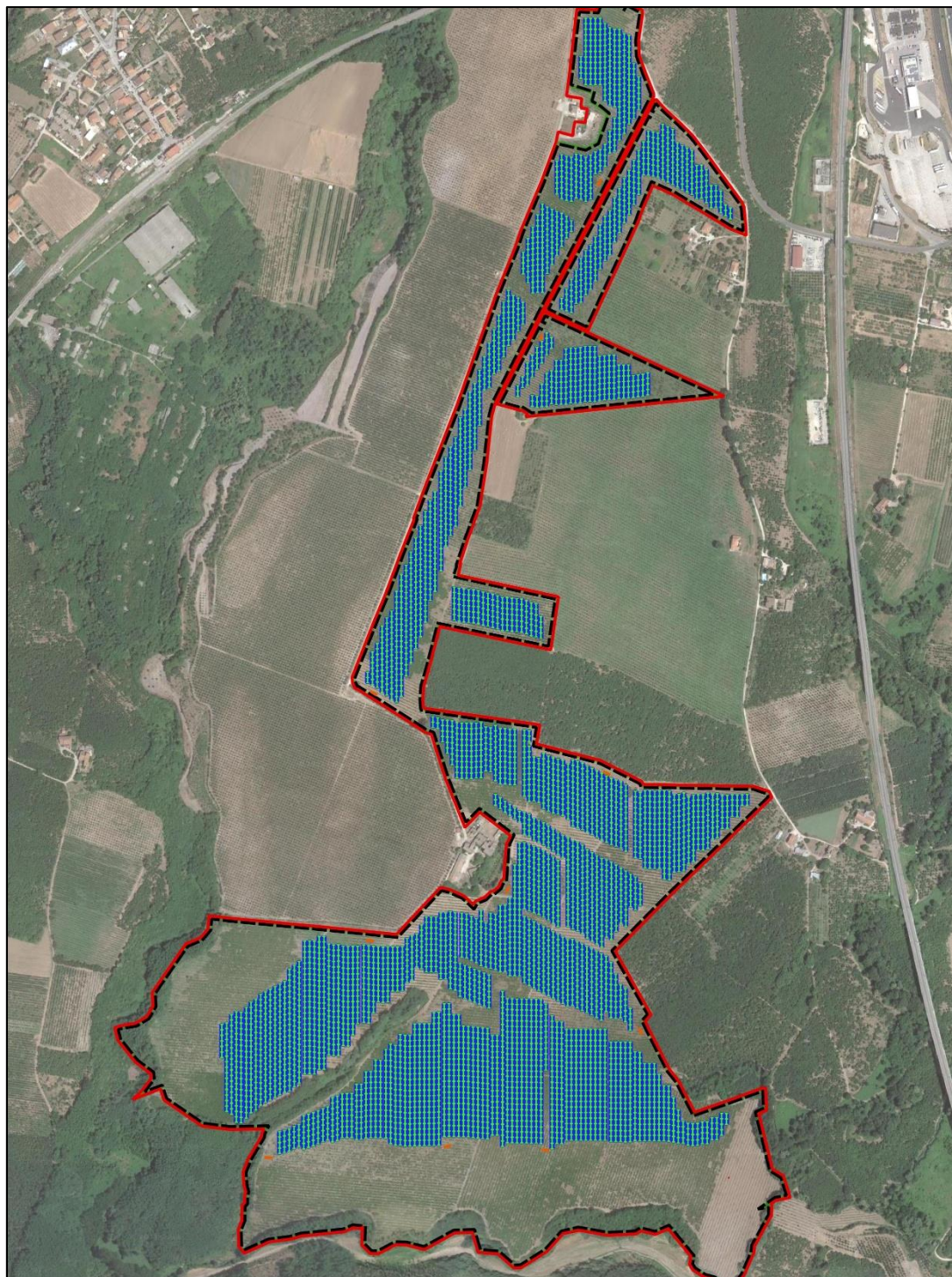
Figura 6 – Planimetria dell'impianto su base ortofoto
