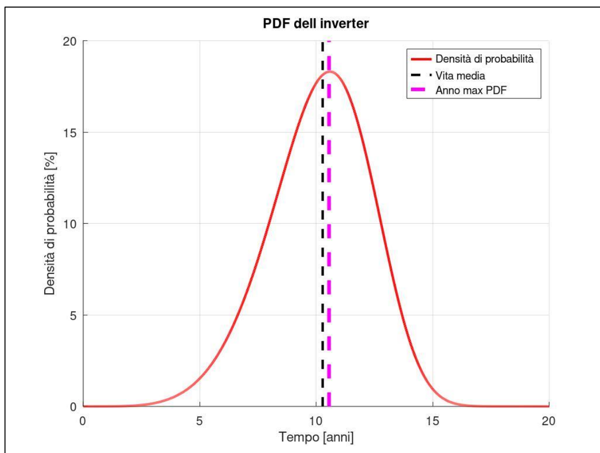
Figura 3 PDF dell'inverter
