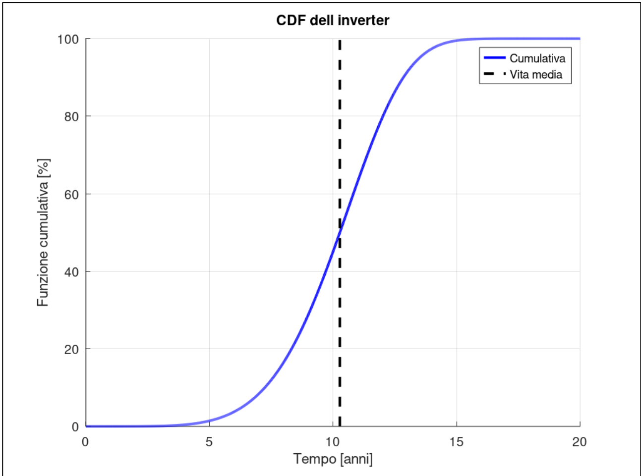
Figura 4 CDF dell'inverter
