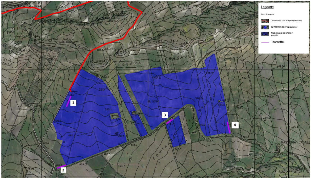
Figura 3 - Inquadramento delle opere di progetto su ortofoto con indicazione dei transetti
