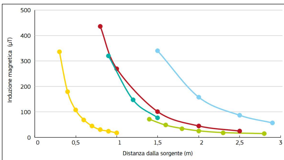
Figura 2: Riduzione dell'induzione magnetica in funzione della distanza per varie sorgenti di frequenza elettrica: saldatrice a punti (—); bobina di smagnetizzazione 0,5 m (—); forno a induzione 180 kW (—); macchina per saldatura continua 100 kVA (—); bobina di smagnetizzazione 1 m (—)
