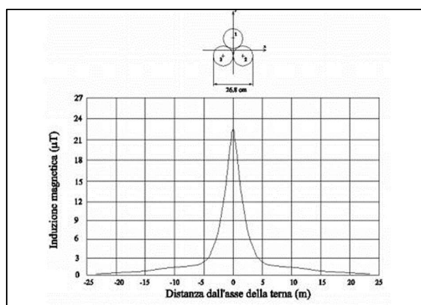
Figura 4: Induzione magnetica al suolo generata da tre cavi disposti a trifoglio
