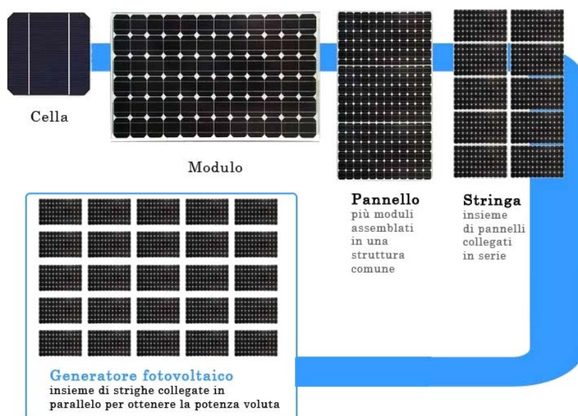
Figura 2. Unità elementari del generatore fotovoltaico
