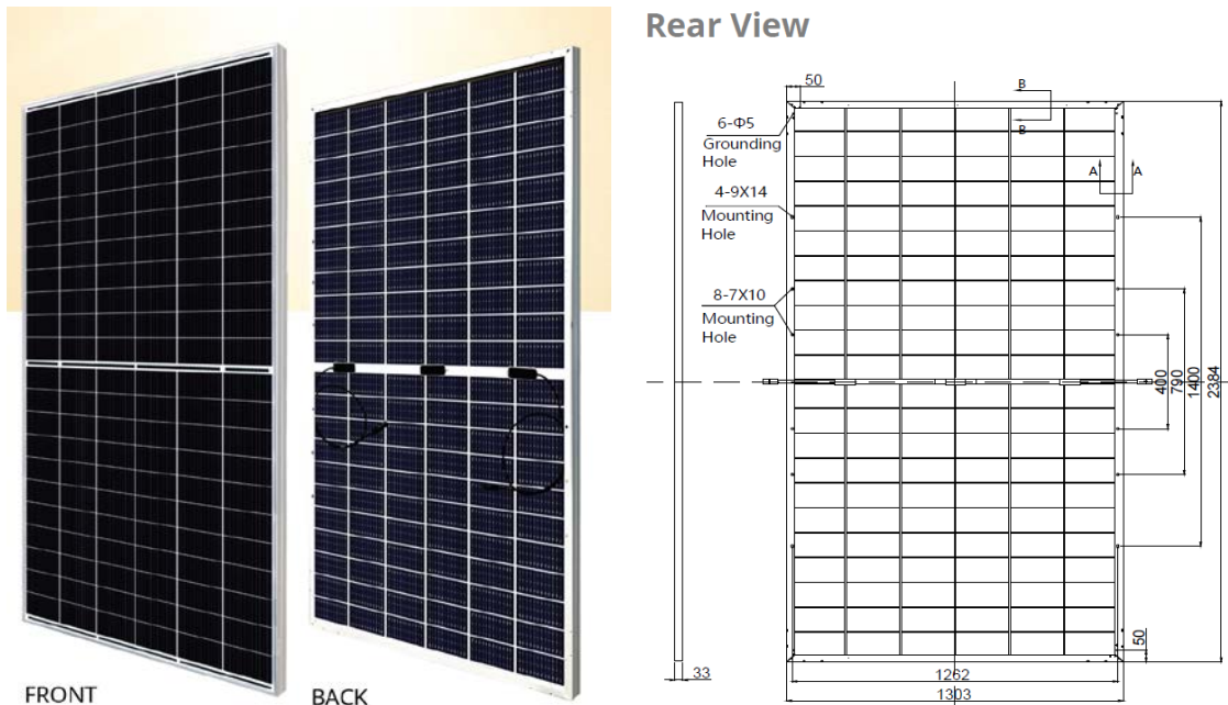
Figura 3. Pannello FV fino a 665 Wp con dimensioni 2384 x 1303 x 35 mm esempio
