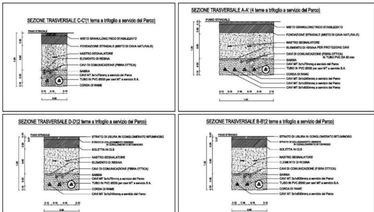
Figura 7. Differenti tipologie di posa del cavidotto
