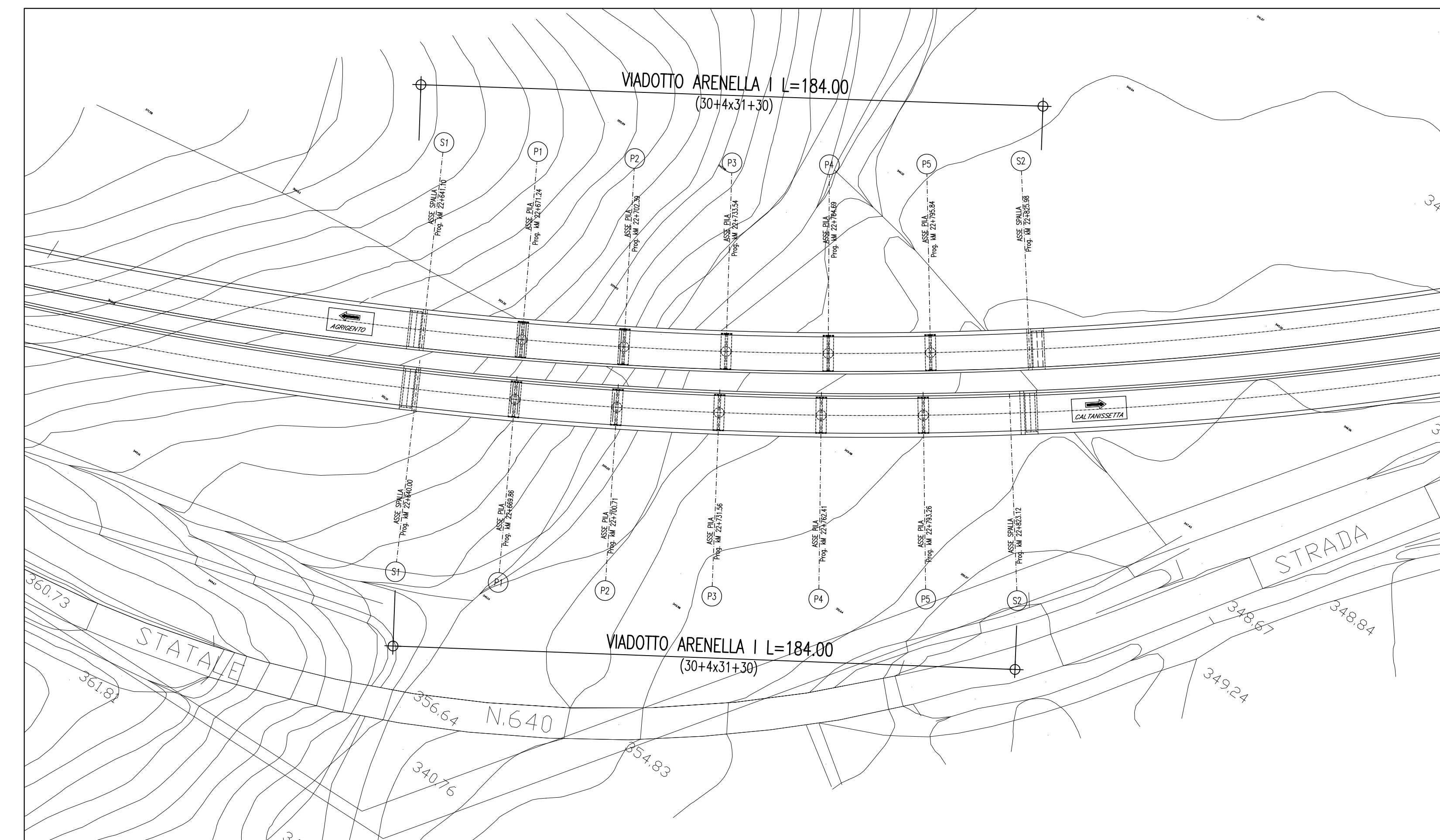
PLANIMETRIA SCALA 1 : 1000
