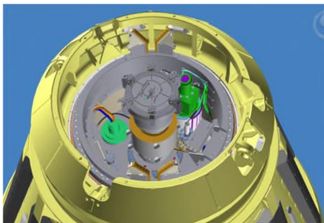
Figura 5-12 Tipico della parte superiore della turret buoy che include il riser e la Stack Valve
