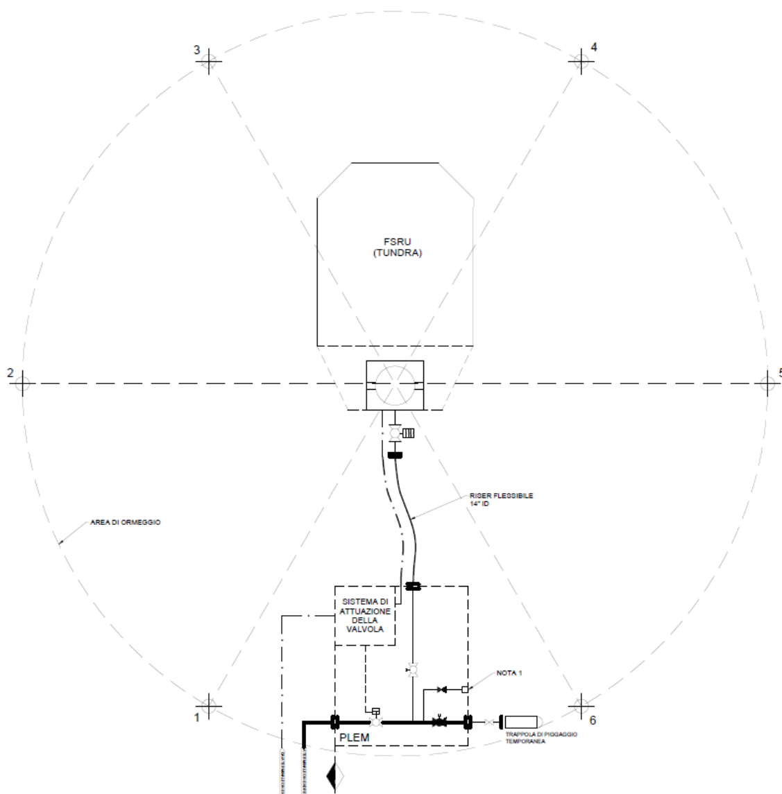
Figura 5-17 Schematico Generale
