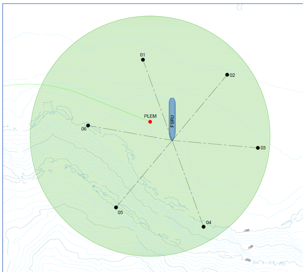
Figura 5-3 Schema di Ormeggio
