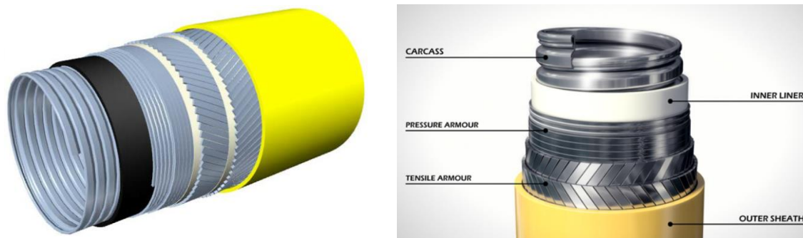
Figura 5-14 Sezione tipica di riser flessibile
