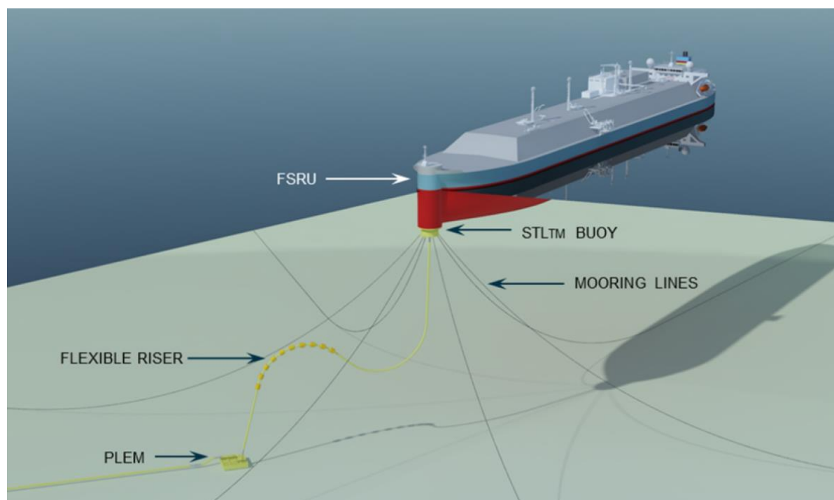
Figura 5-15 Schema (tipico) del sistema di ormeggio
