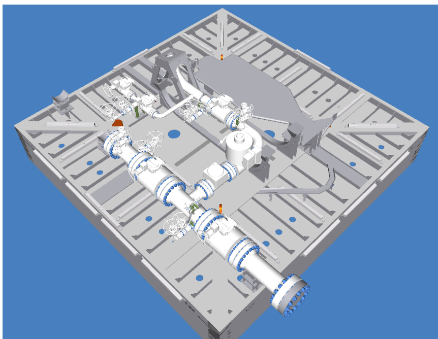
Figura 5-16 Tipica configurazione del PLEM
