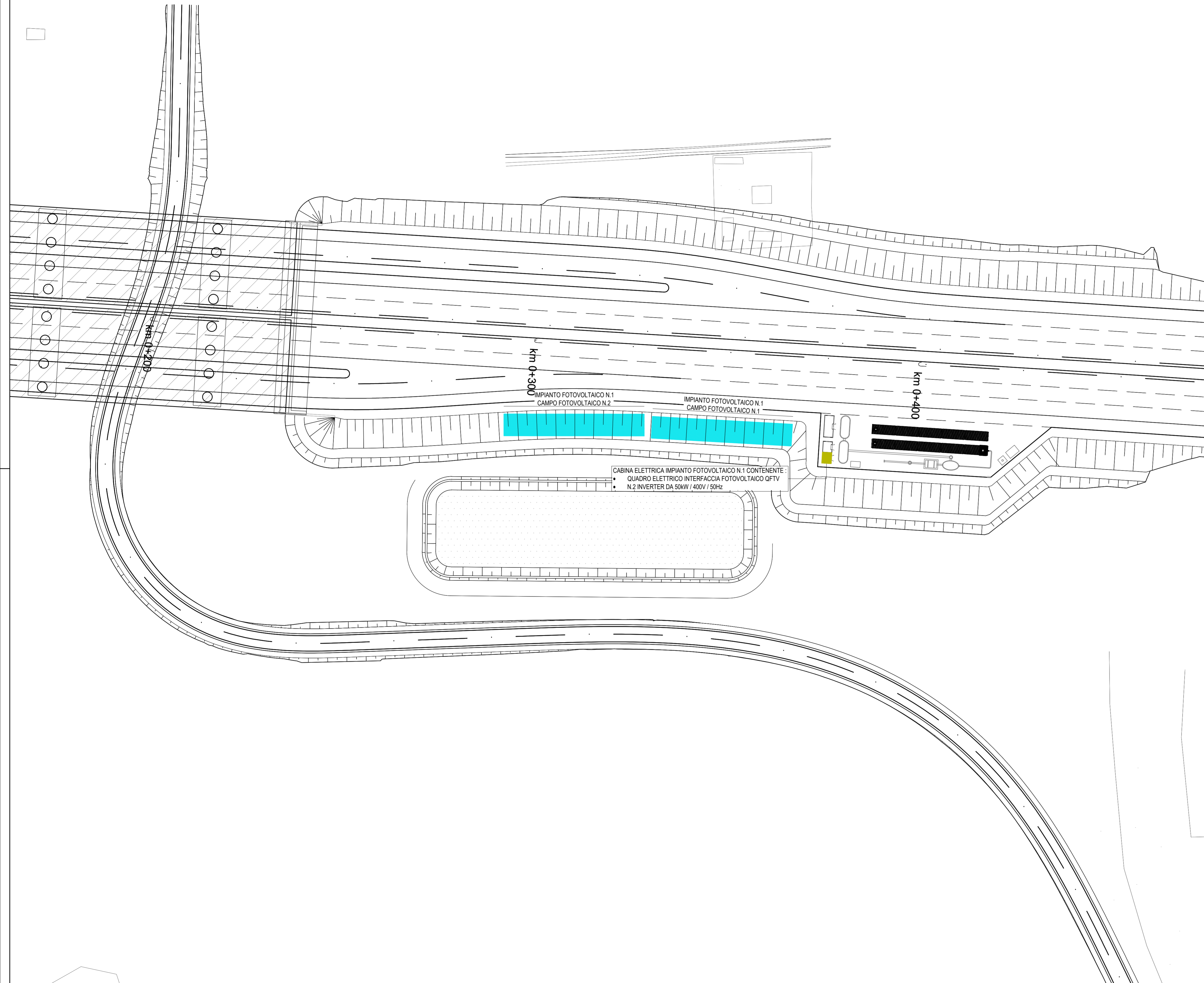
PLANIMETRIA CON UBICAZIONE IMPIANTO FOTOVOLTAICO N.1 Scala 1:500
