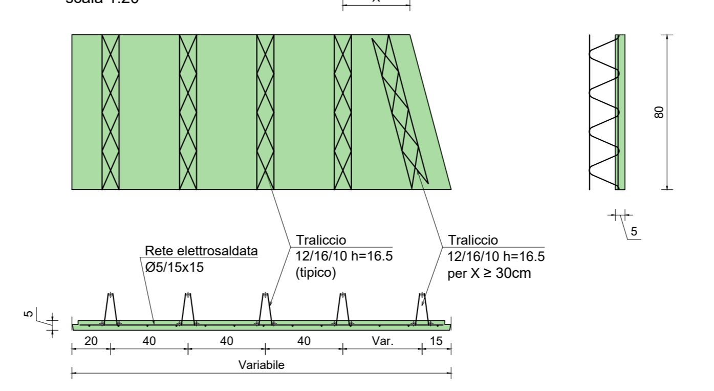
PREDALLA TIPO -Bs- scala 1:20
