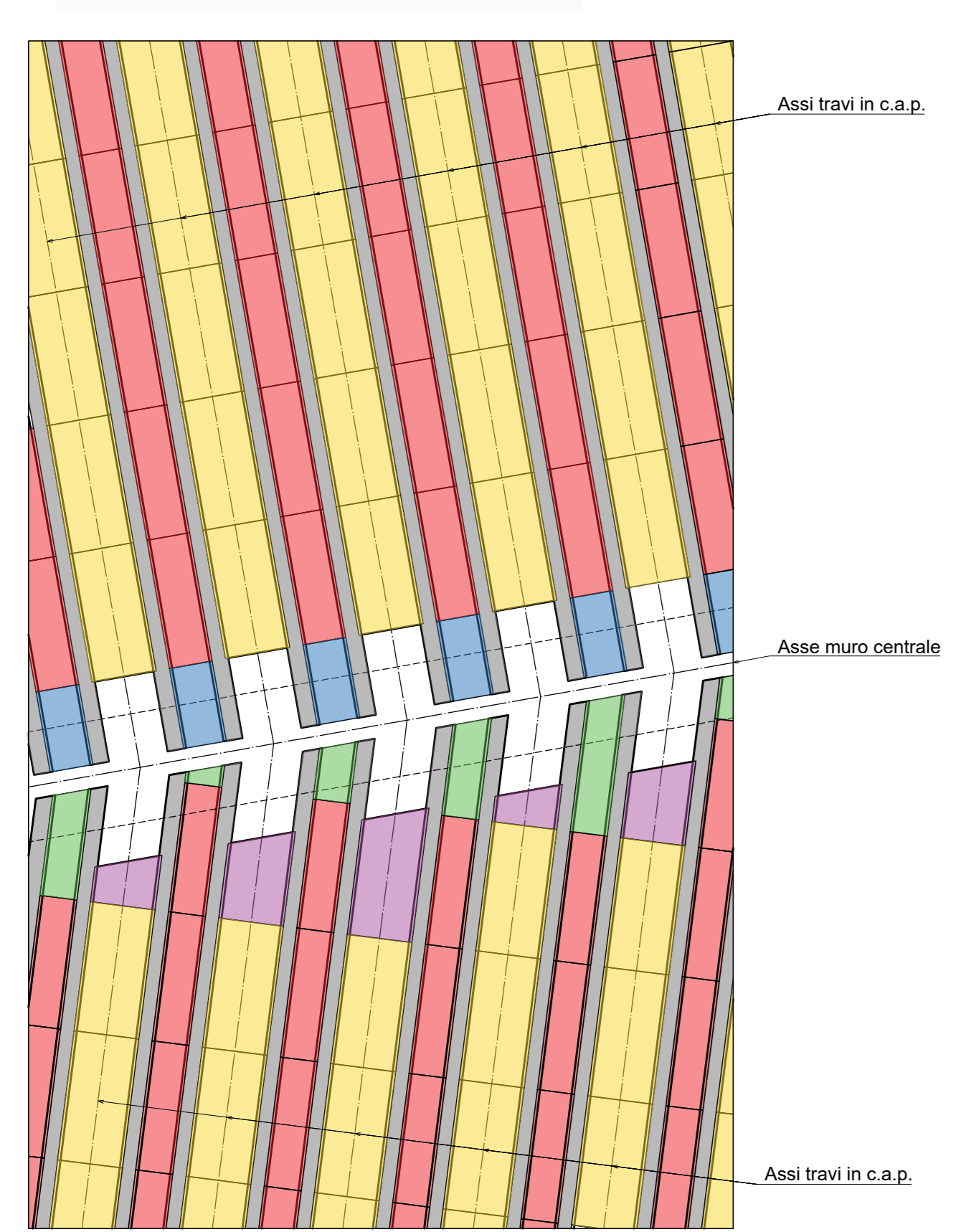
STRALCIO IMPALCATO TIPOLOGIA PREDALLE scala 1:100
