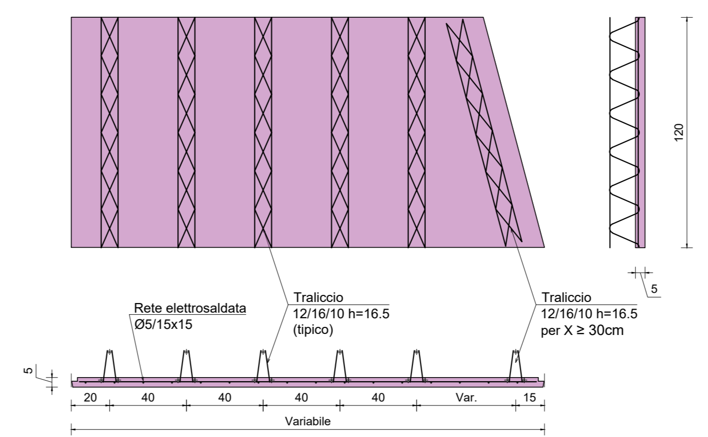
PREDALLA TIPO -Bs- scala 1:20
