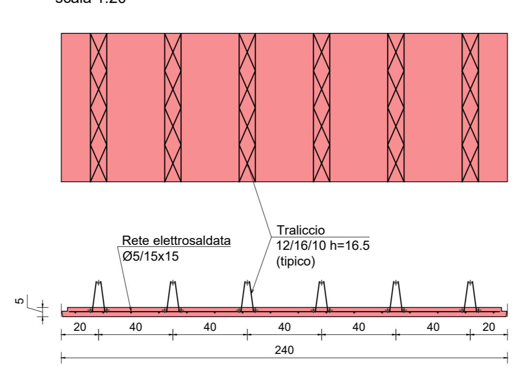
PREDALLA TIPO -B- scala 1:20
