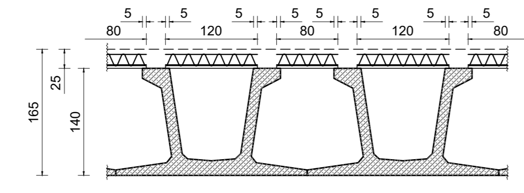
STRALCIO SEZIONE TRASVERSALE IMPALCATO DISPOSIZIONE PREDALLE scala 1:50
