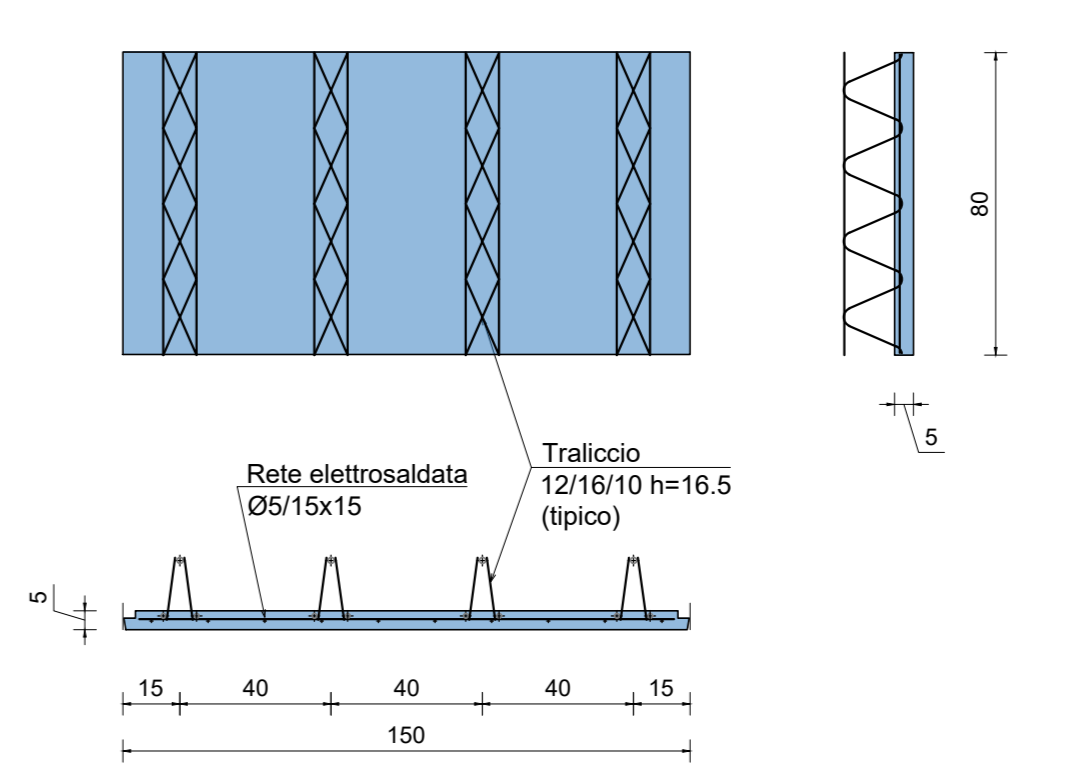
PREDALLA TIPO -C- scala 1:20
