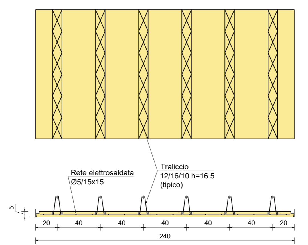
PREDALLA TIPO -B- scala 1:20
