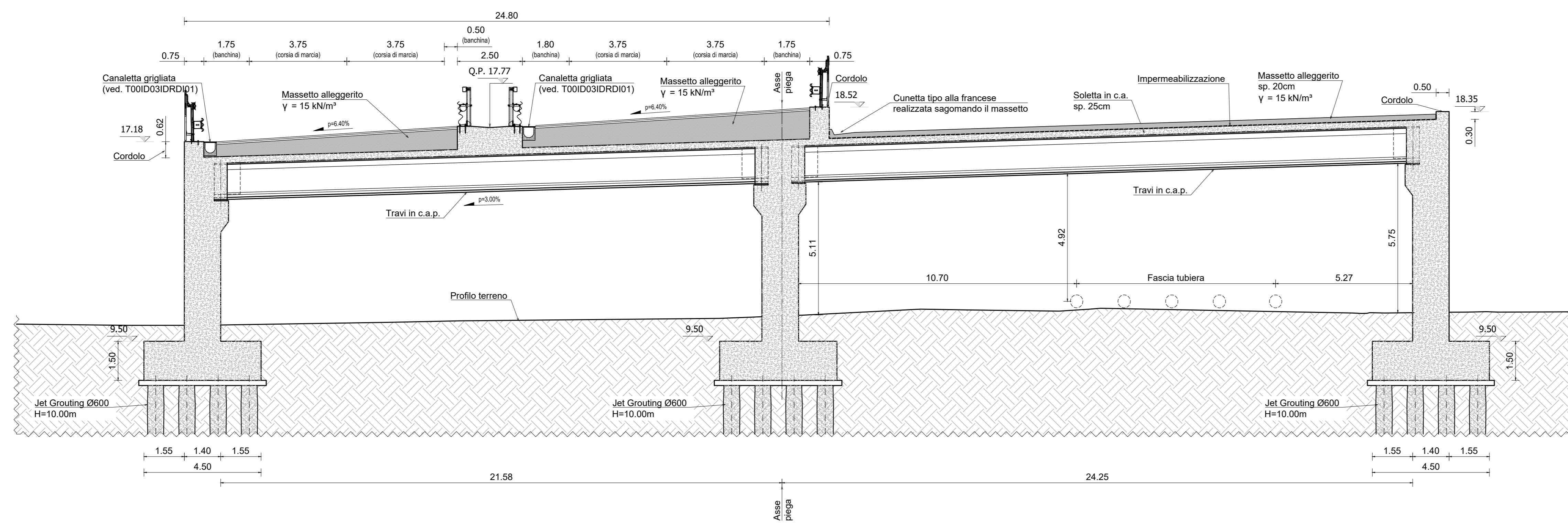
SEZIONE A-A scala 1:100
