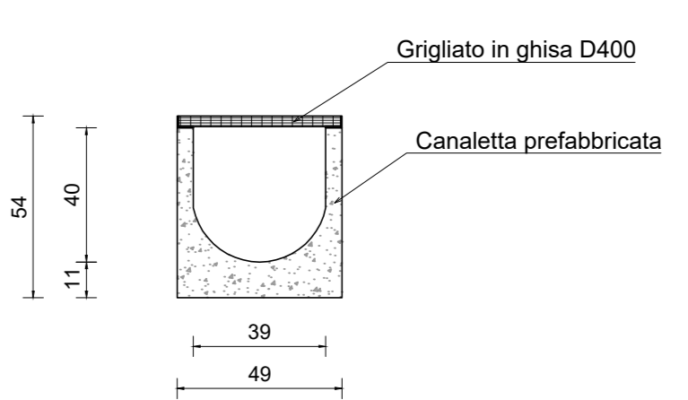
PARTICOLARE CANALETTA PREFABBRICATA PER RACCOLTA ACQUE DI PIATTAFORMA STRADALE scala 1:20
