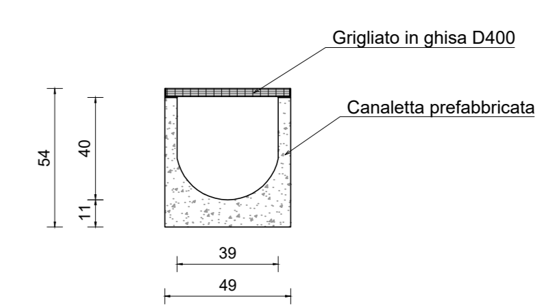
PARTICOLARE CANALETTA PREFABBRICATA PER RACCOLTA ACQUE DI PIATTAFORMA STRADALE scala 1:20
