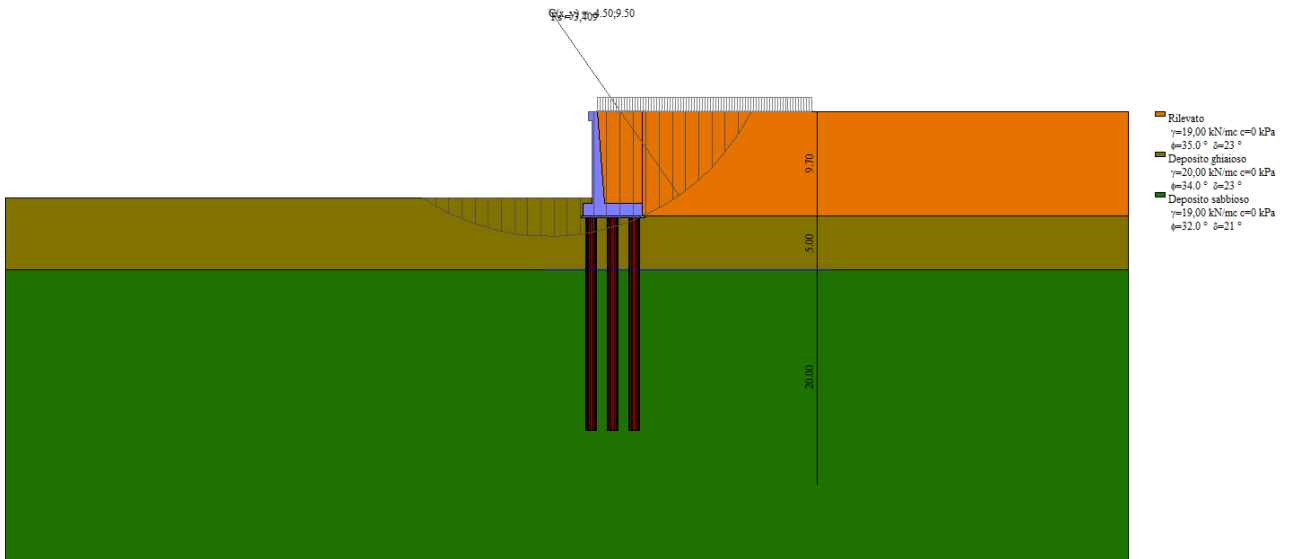
Figura 8-25. Analisi stabilità – Combinazione piu sfavorevole (Comb. 5) – FS=3.41
