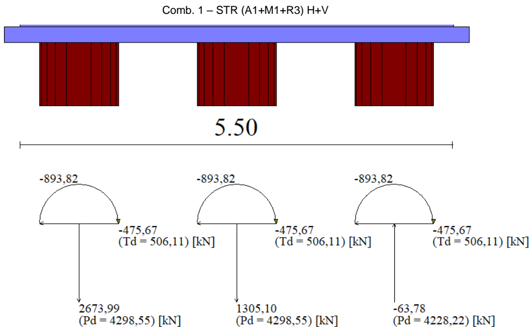
Figura 8-13: Scarichi in testa ai pali di fondazione del muro per la combinazione più sfavorevole (Comb.1)
