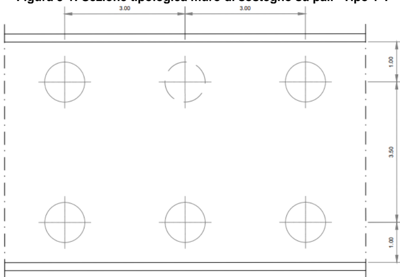
Figura 5-2: Pianta muro di sostegno su pali "Tipo 1".
