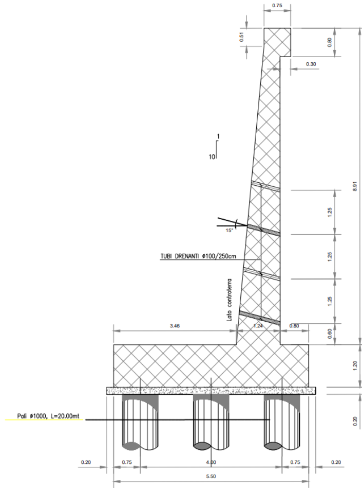
Figura 5-3: Sezione tipologica muro di sostegno su pali "Tipo 2".
