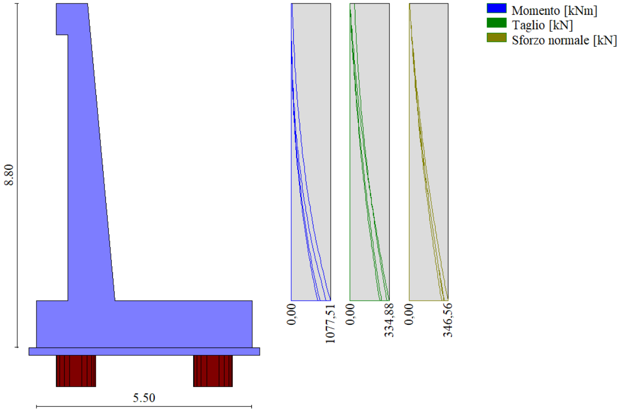
Figura 8-1: Involuppo delle sollecitazioni del paramento del muro
