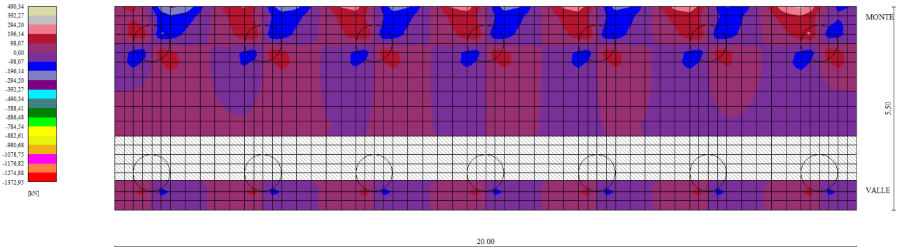
Figura 8-4: Txx sulla fondazione del muro – Comb.2 - |T_{xx,max}|=254 kN
