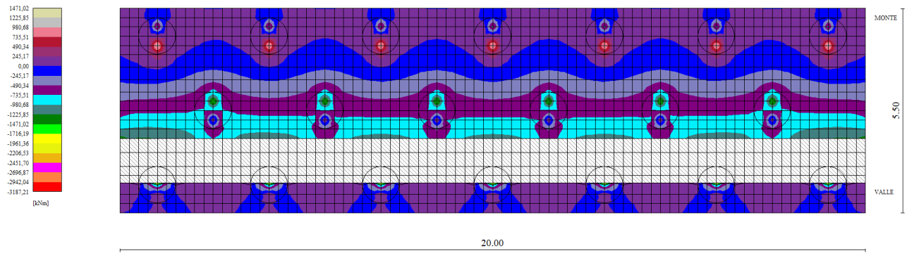
Figura 8-10: Myy sulla fondazione del muro – Comb. 2 – Myy,max = 1320 kN
