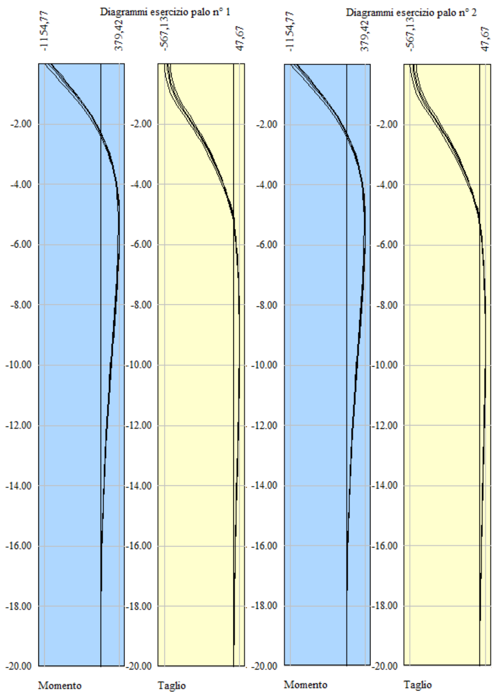
Figura 8-7: Involuppo delle sollecitazioni flettenti e taglianti lungo i pali di fondazione.
