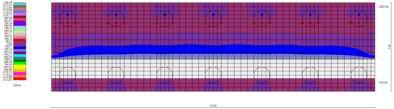
Figura 8-2: Mxx sulla fondazione dei muri – Comb. 2 – Mxx,max = 264.5 kN
