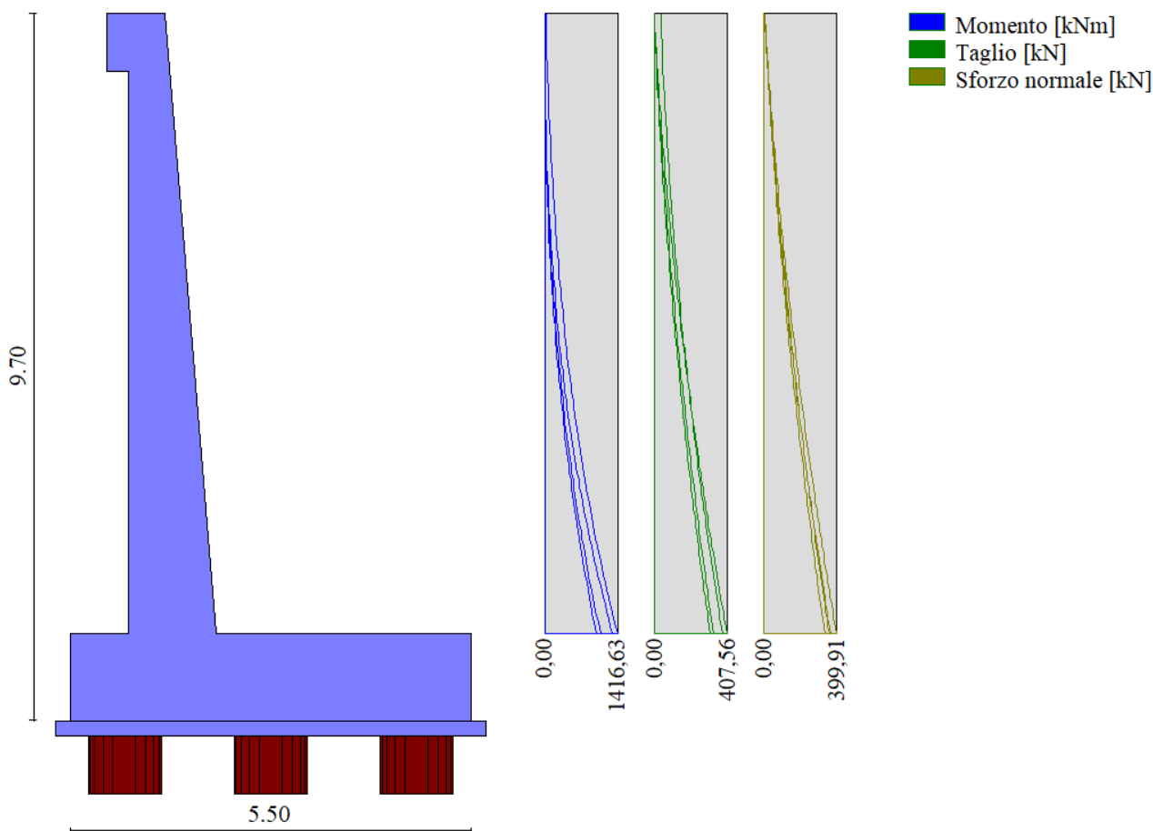
Figura 8-8: Involuppo delle sollecitazioni del paramento del muro
