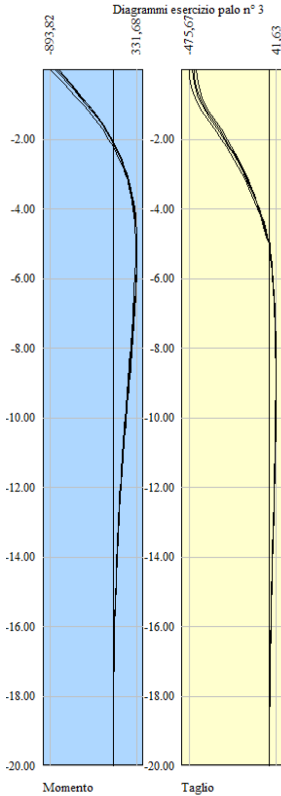
Figura 8-15: Involuppo delle sollecitazioni flettenti e taglianti lungo i pali di fondazione (fila 3).
