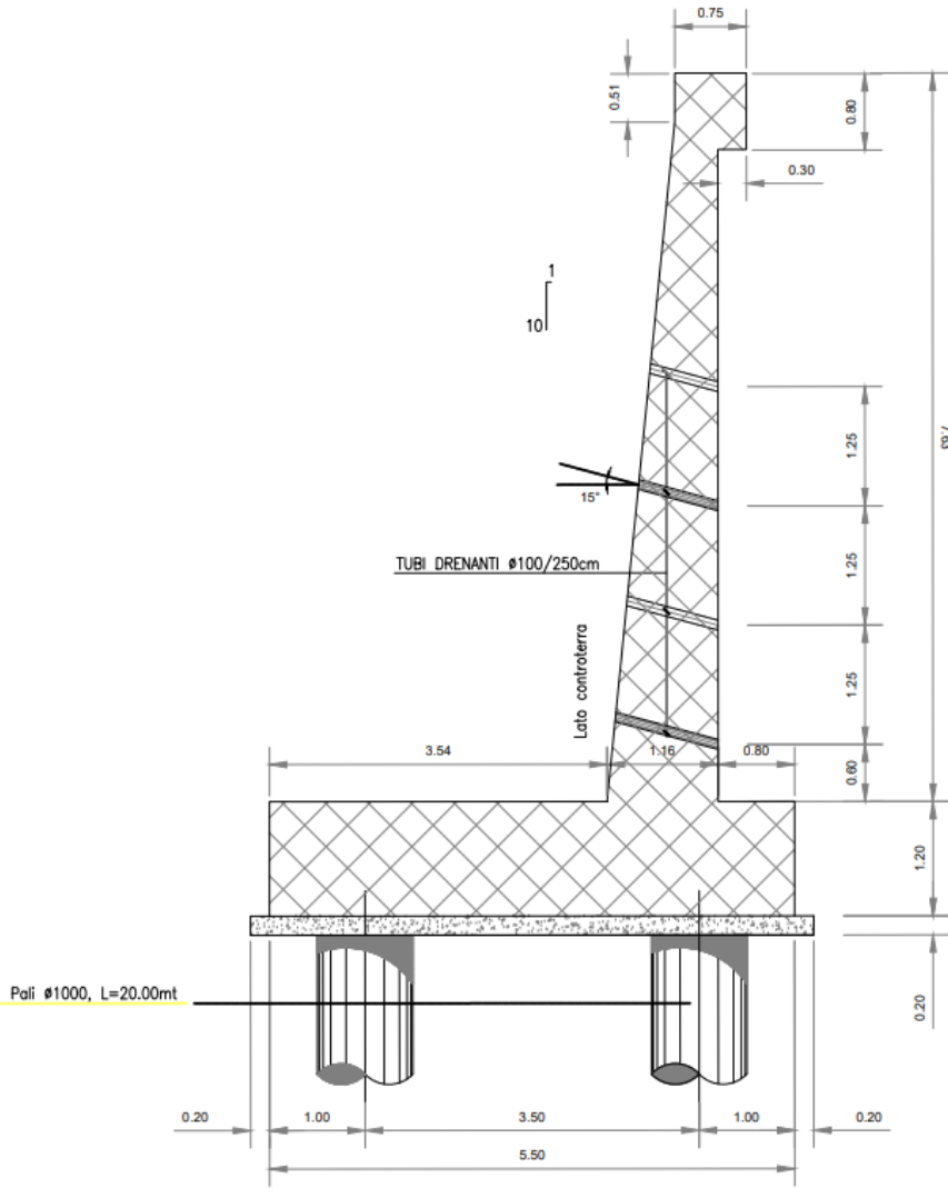
Figura 5-1: Sezione tipologica muro di sostegno su pali "Tipo 1".
