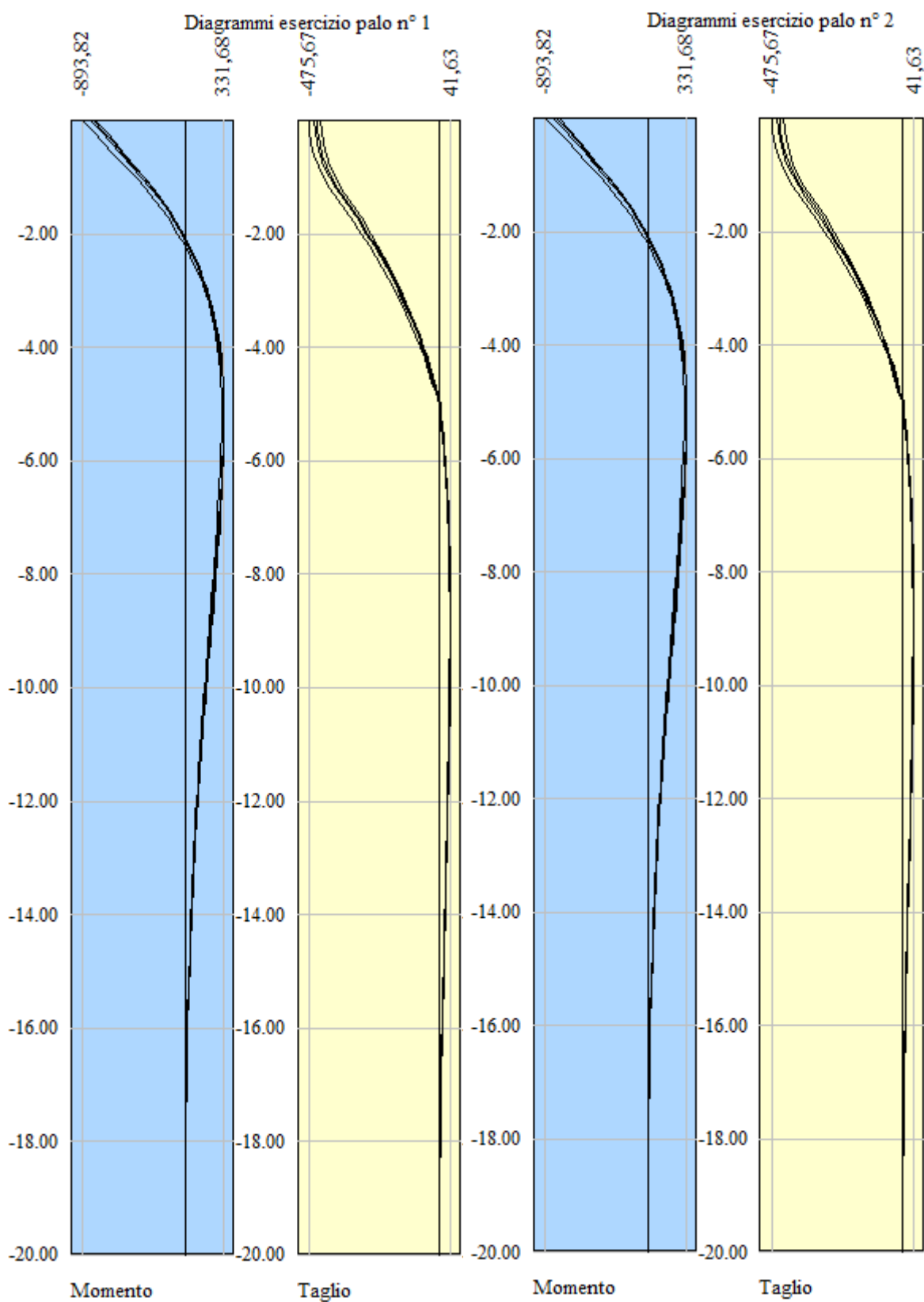
Figura 8-14: Involuppo delle sollecitazioni flettenti e taglianti lungo i pali di fondazione (fila 1 e fila 2).
