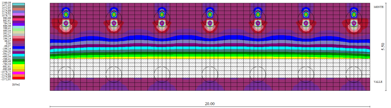
Figura 8-3: Myy sulla fondazione del muro – Comb. 2 – Myy,max = 882.6 kN
