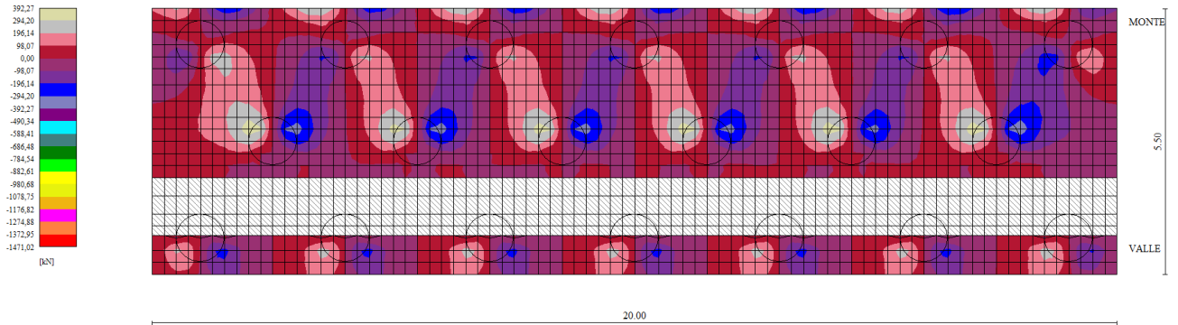
Figura 8-11: Txx sulla fondazione del muro – Comb.2 - |T_{xx,max}|=342 kN
