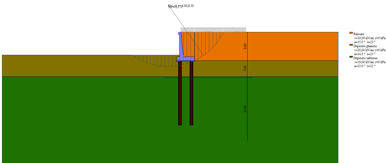
Figura 8-24. Analisi stabilità – Combinazione piu sfavorevole (Comb. 5) – FS=3.17
