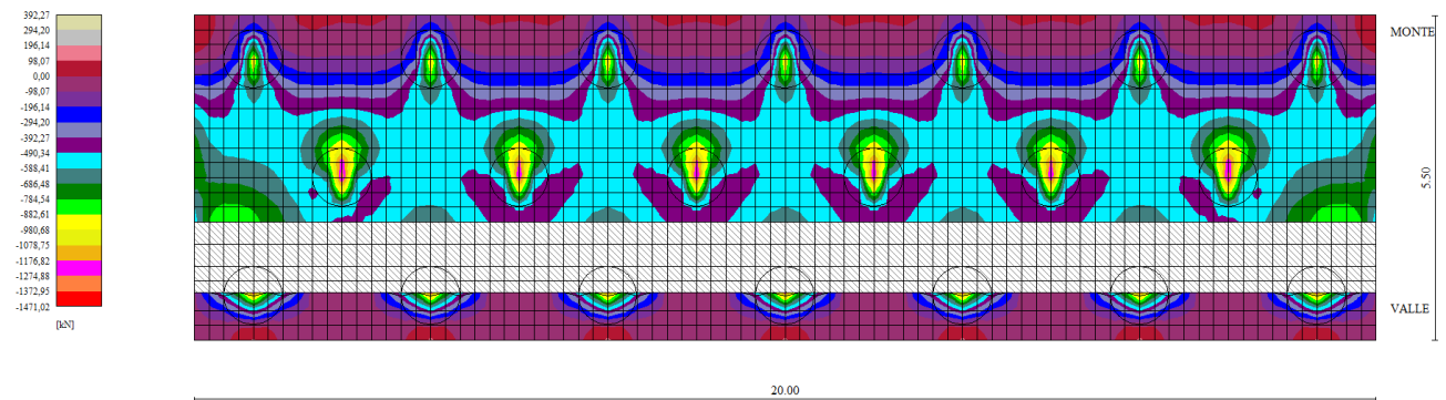
Figura 8-12: Tyy sulla fondazione del muro – Comb.2 - |T_{yy,max}|=841 kN
