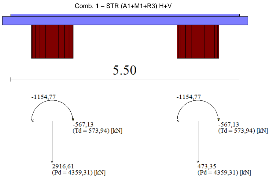
Figura 8-6: Scarichi in testa ai pali di fondazione del muro per la combinazione piu sfavorevole (Comb.1)
