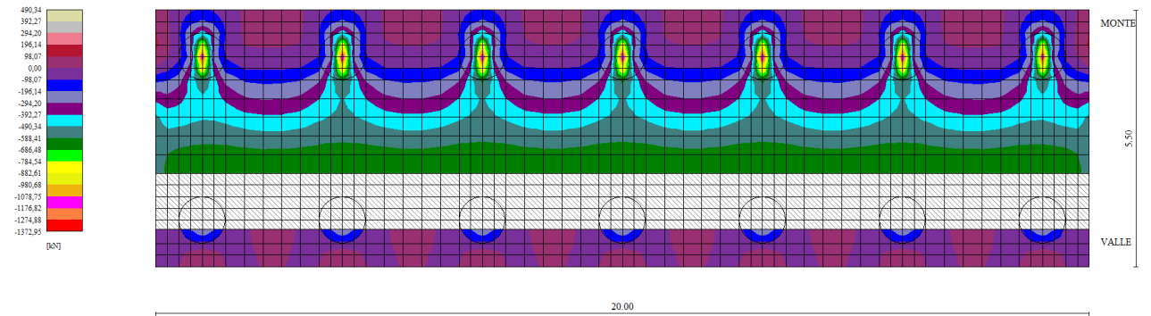
Figura 8-5: Tyy sulla fondazione del muro – Comb.2 - |T_{yy,max}|=681 kN
