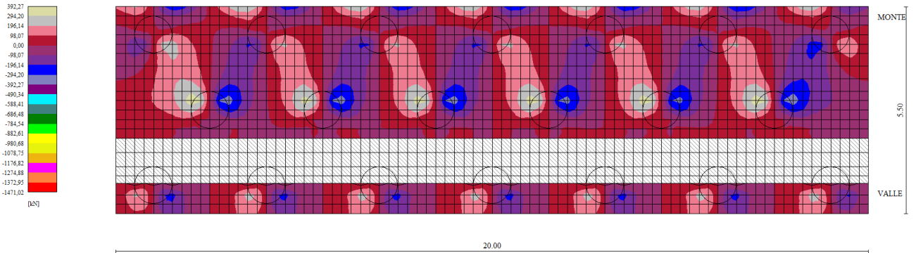
Figura 8-4: Txx sulla fondazione del muro – Comb.2 - |T_{xx,max}|=342 kN
