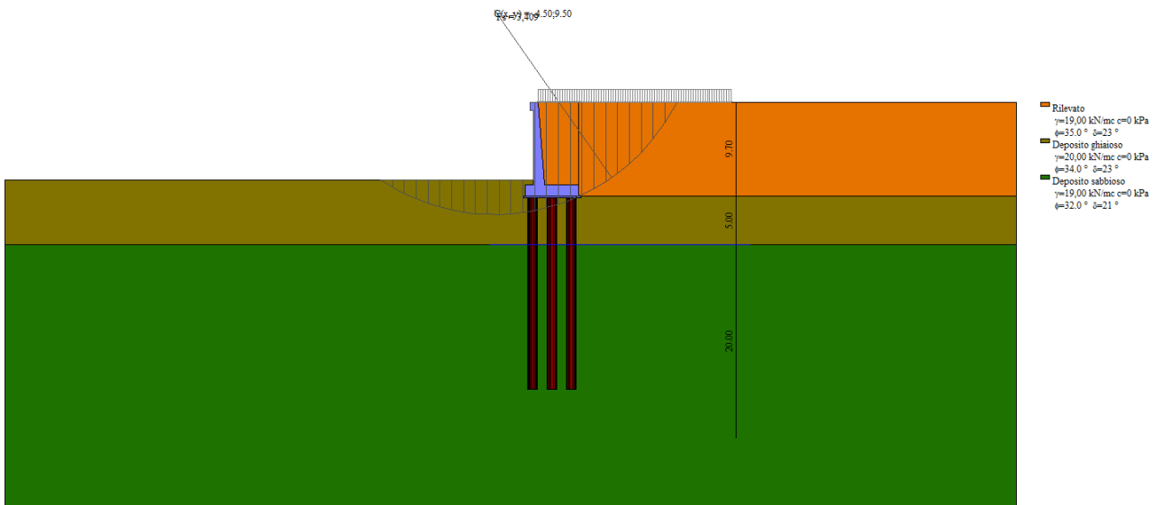
Figura 8-13. Analisi stabilità – Combinazione piu sfavorevole (Comb. 5) – FS=3.41
