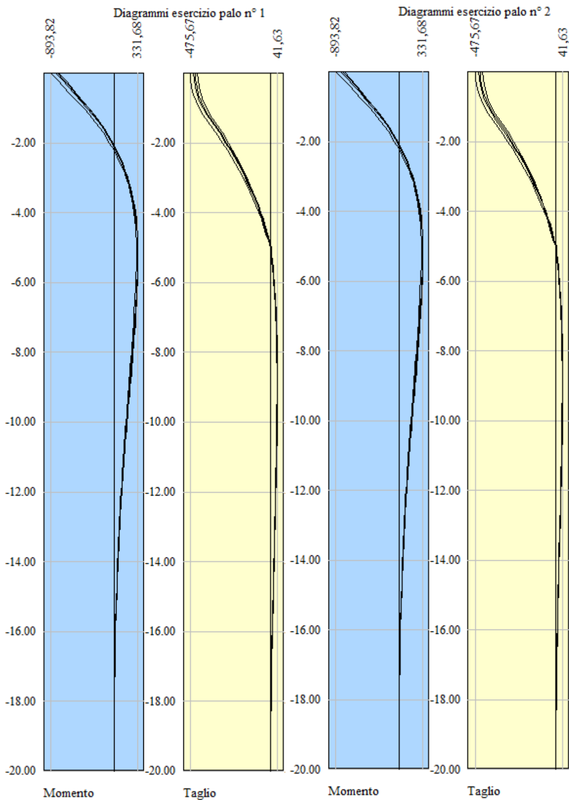
Figura 8-7: Involuppo delle sollecitazioni flettenti e taglianti lungo i pali di fondazione (fila 1 e fila 2).
