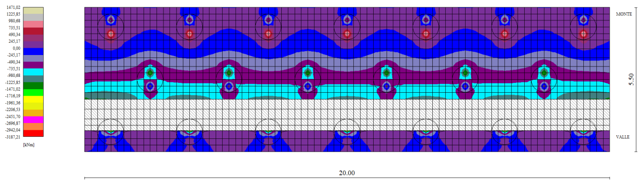
Figura 8-3: Myy sulla fondazione del muro – Comb. 2 – Myy,max = 1320 kN
