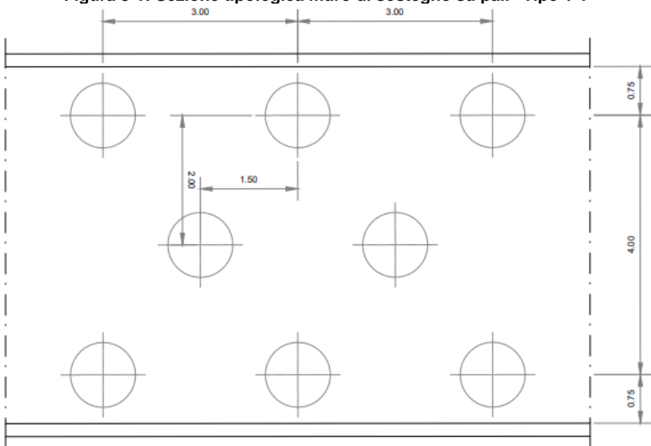
Figura 5-1: Sezione tipologica muro di sostegno su pali "Tipo 1".
