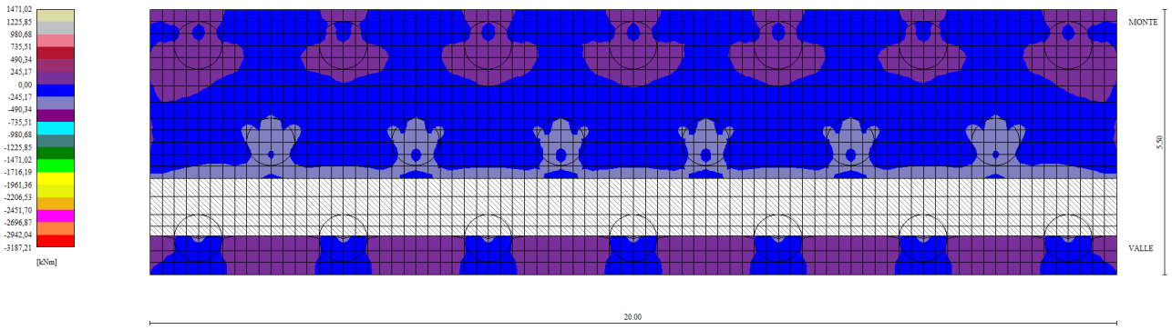
Figura 8-2: Mxx sulla fondazione dei muri – Comb. 2 – Mxx,max = 368 kN
