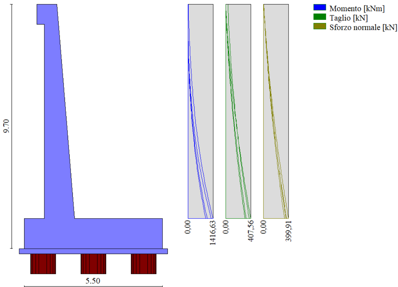
Figura 8-1: Involuppo delle sollecitazioni del paramento del muro
