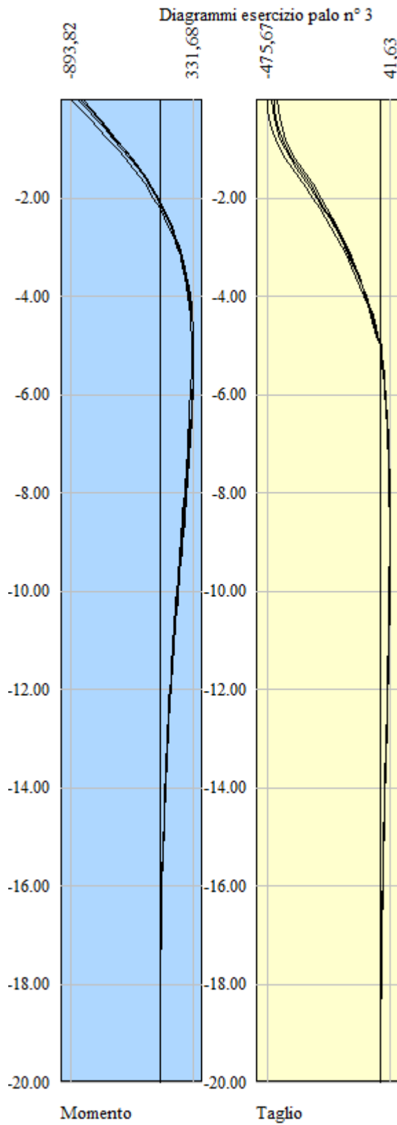
Figura 8-8: Involuppo delle sollecitazioni flettenti e taglianti lungo i pali di fondazione (fila 3).
