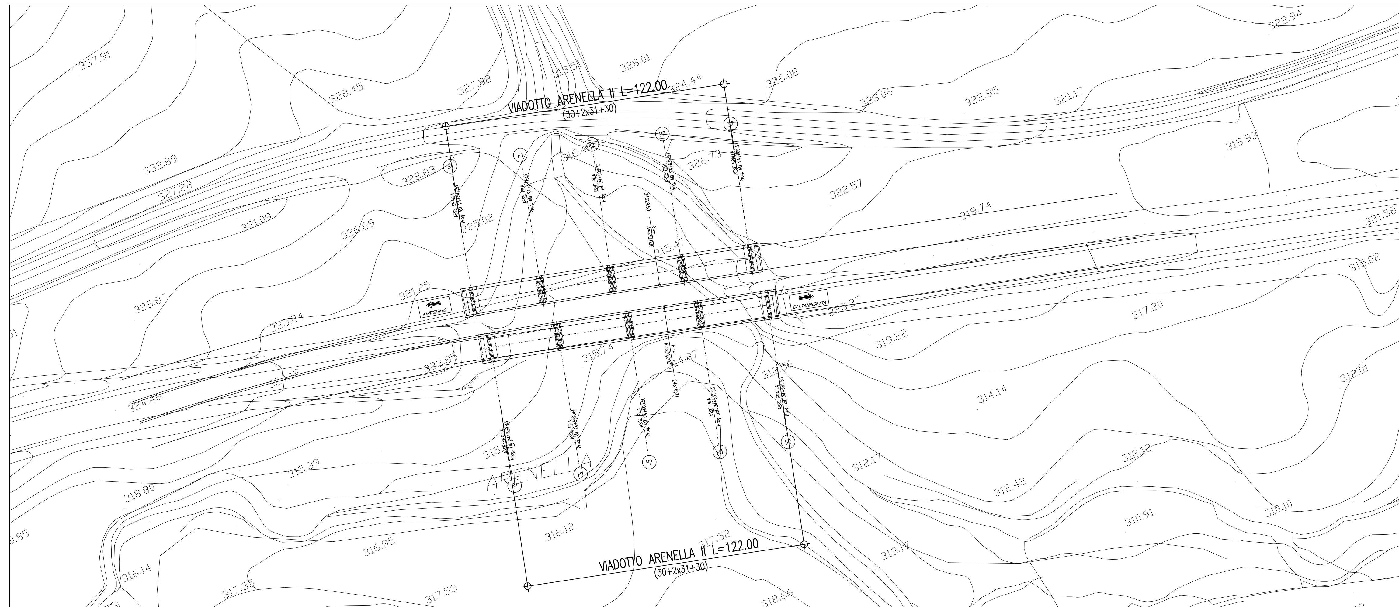
PLANIMETRIA SCALA 1 : 1000
