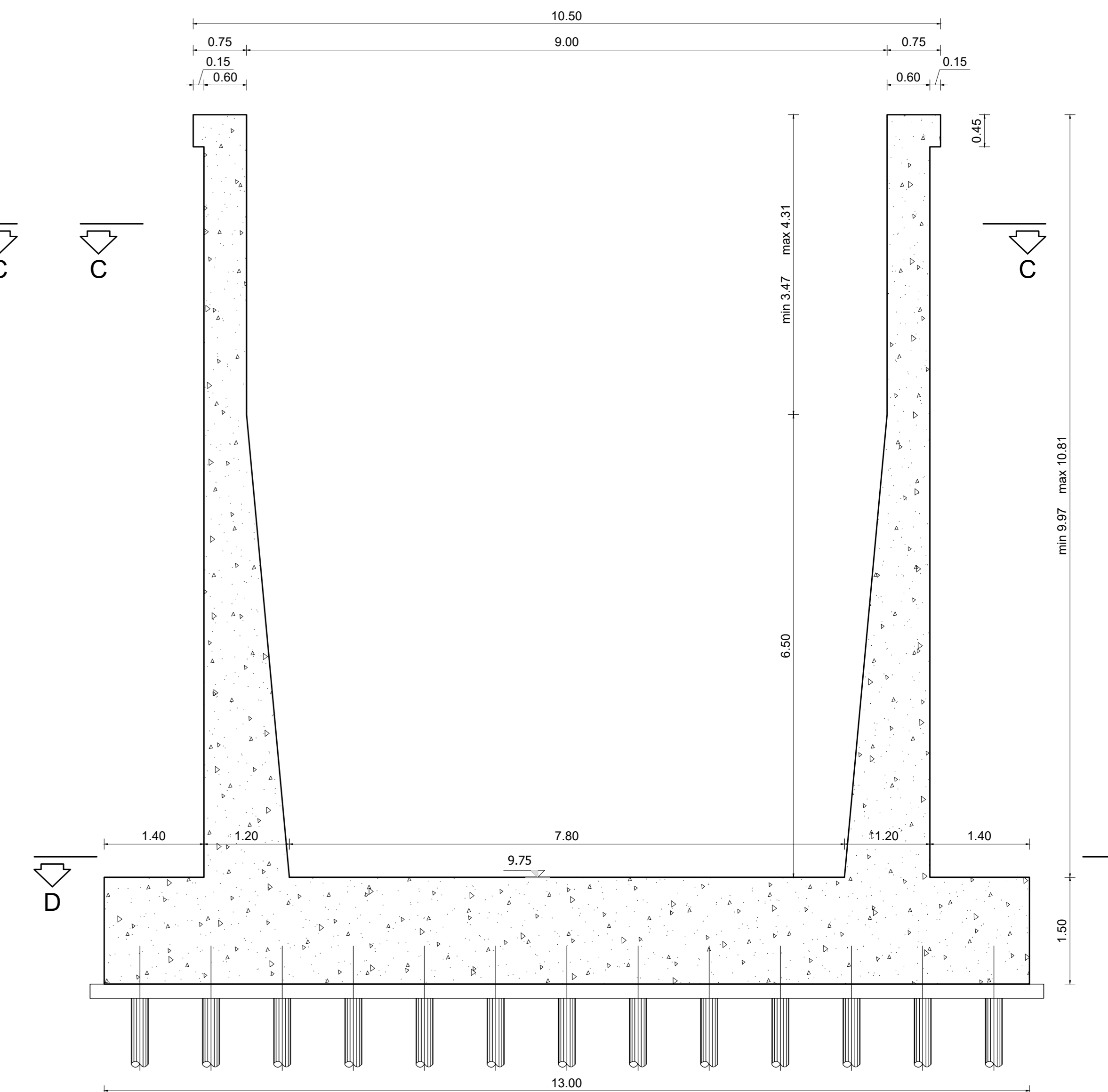
SEZIONE B-B SPALLA "SP2" LATO ROTATORIA 2 scala 1:50
