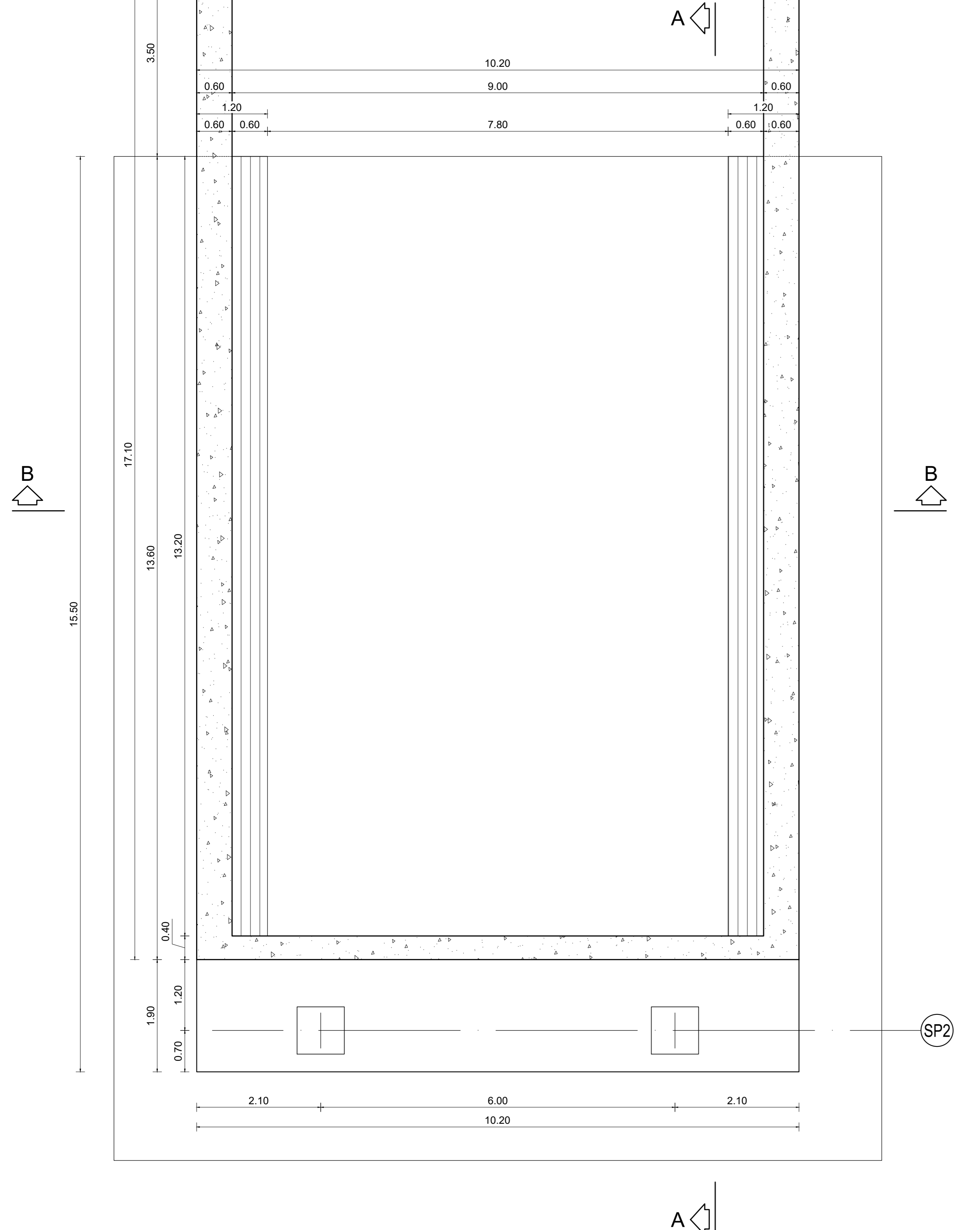
SEZIONE C-C PIANTA APOGGI SPALLA "SP2" LATO ROTATORIA 2 scala 1:50
