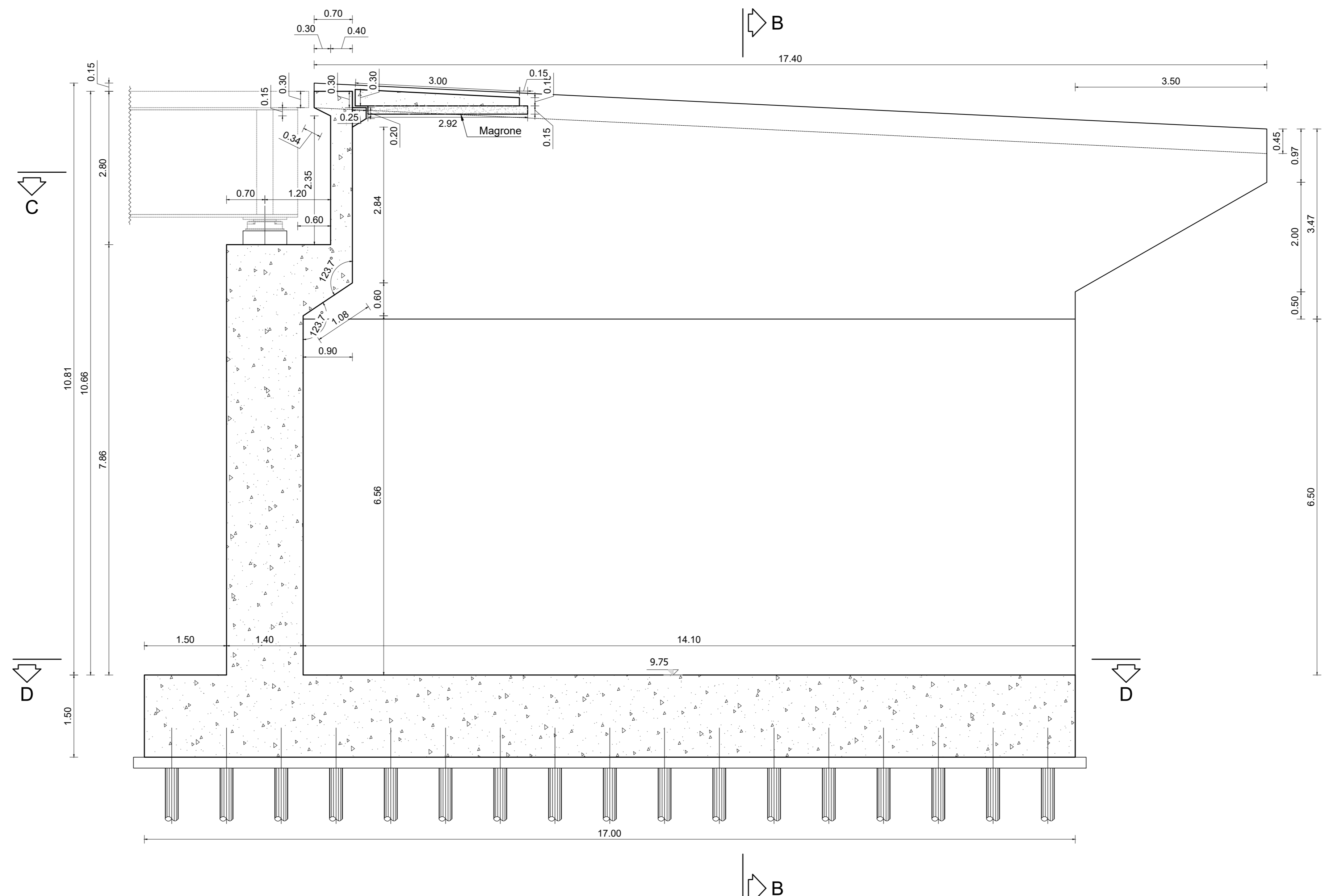
SEZIONE A-A SPALLA "SP2" LATO ROTATORIA 2 scala 1:50
