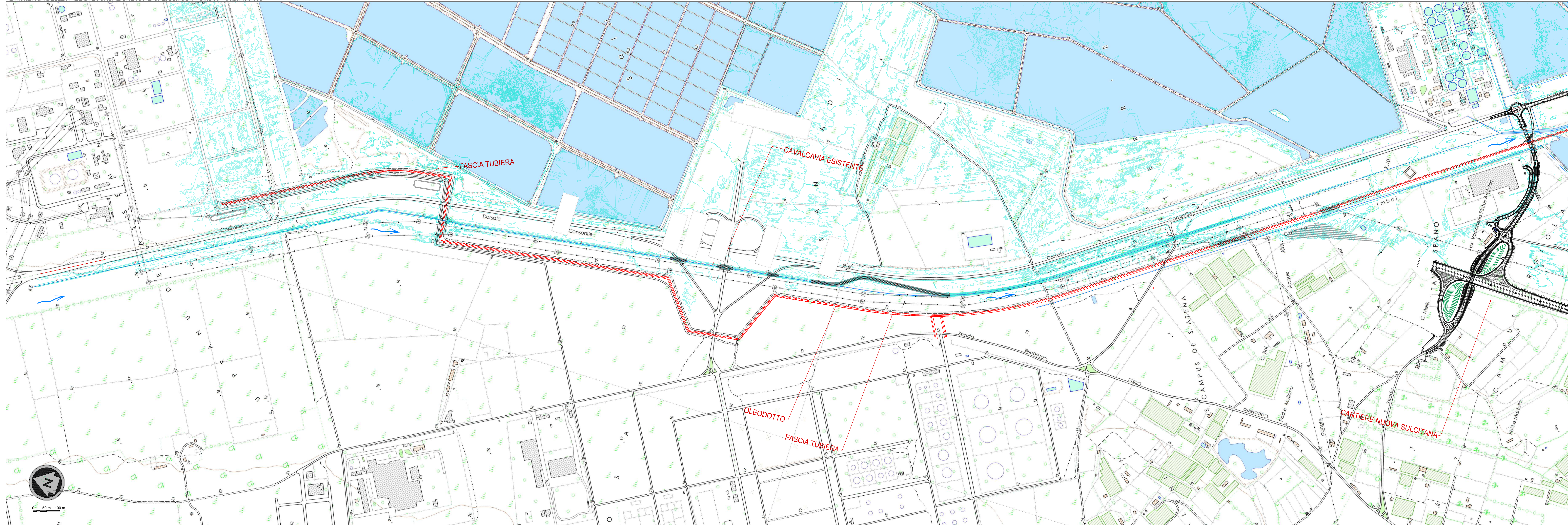
PLANIMETRIA DELLE AREE DI ESONDAZIONE POST OPERAM - Scala 1:5 000
