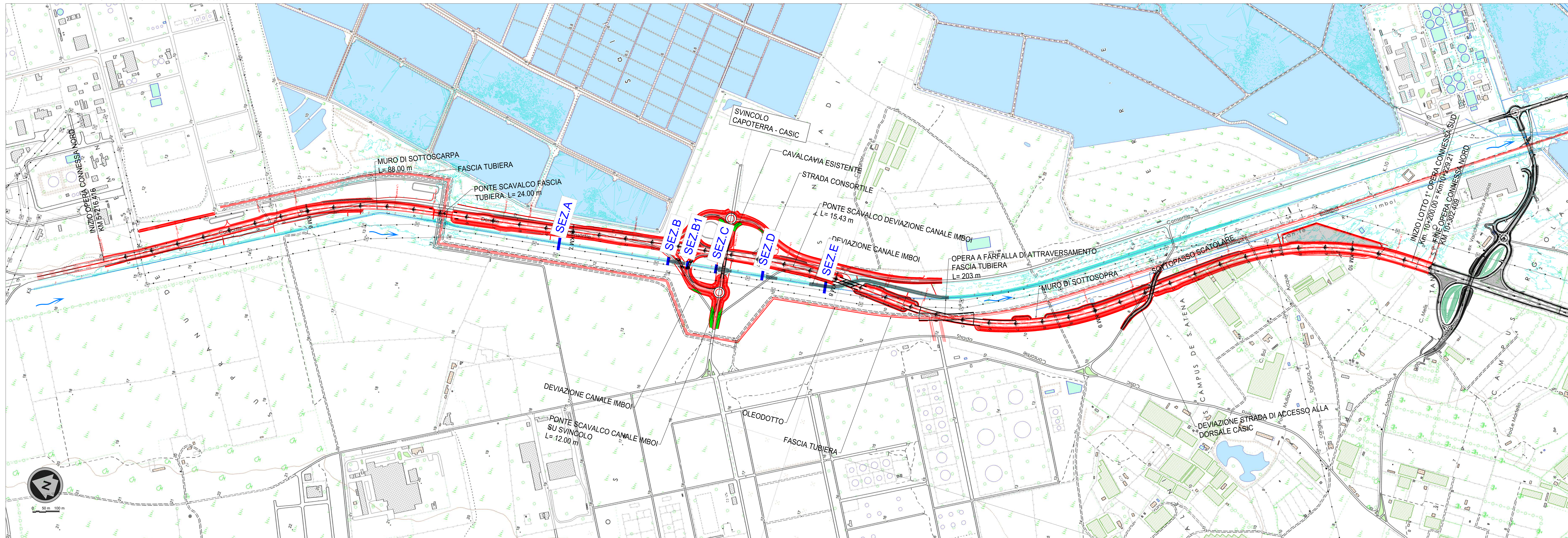
PLANIMETRIA DELLE AREE DI ESONDAZIONE POST OPERAM - Scala 1:5 000
