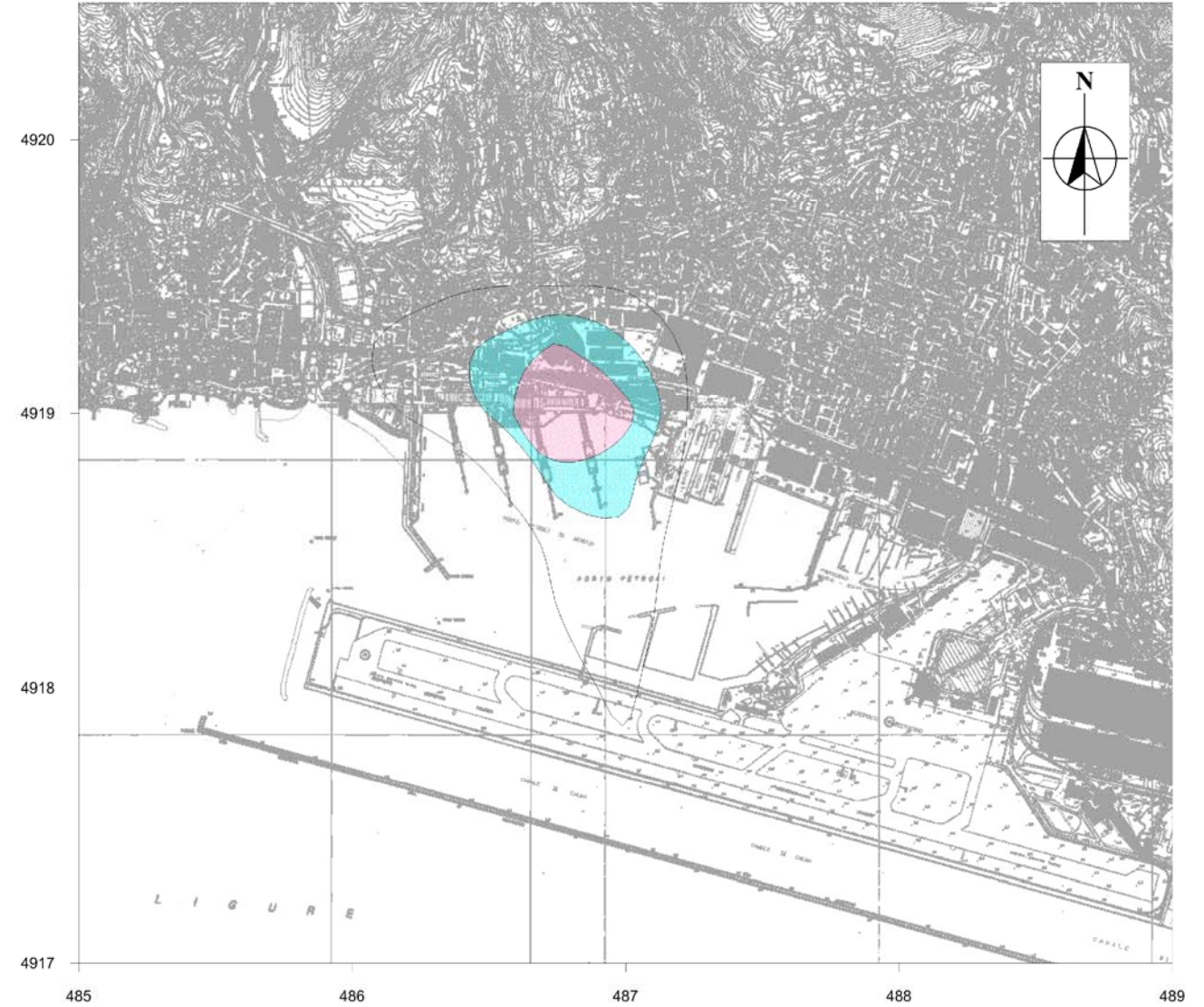
ISOCONCENTRAZIONI DI NOx
