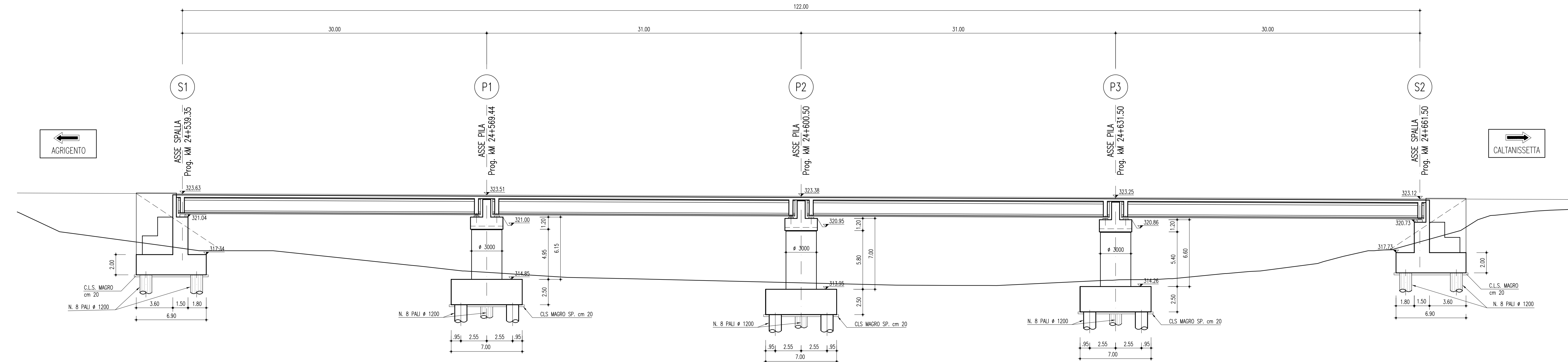
SEZIONE LONGITUDINALE PISTA DESTRA (CALTANISSETTA) SCALA 1 : 200
