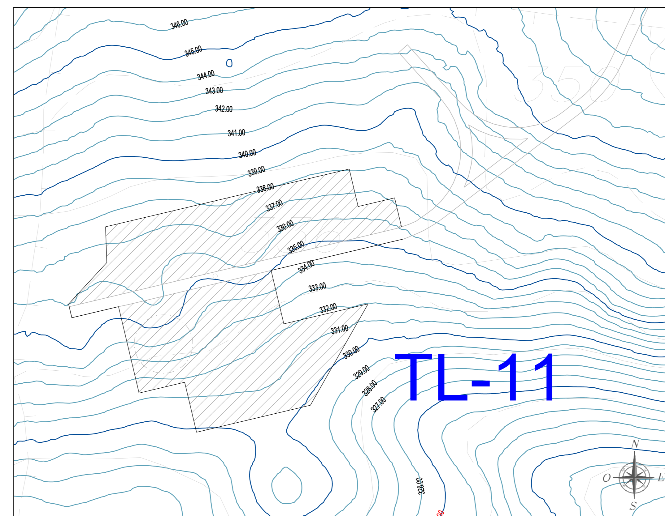
QUADRO 28 - Scala 1:1.000
