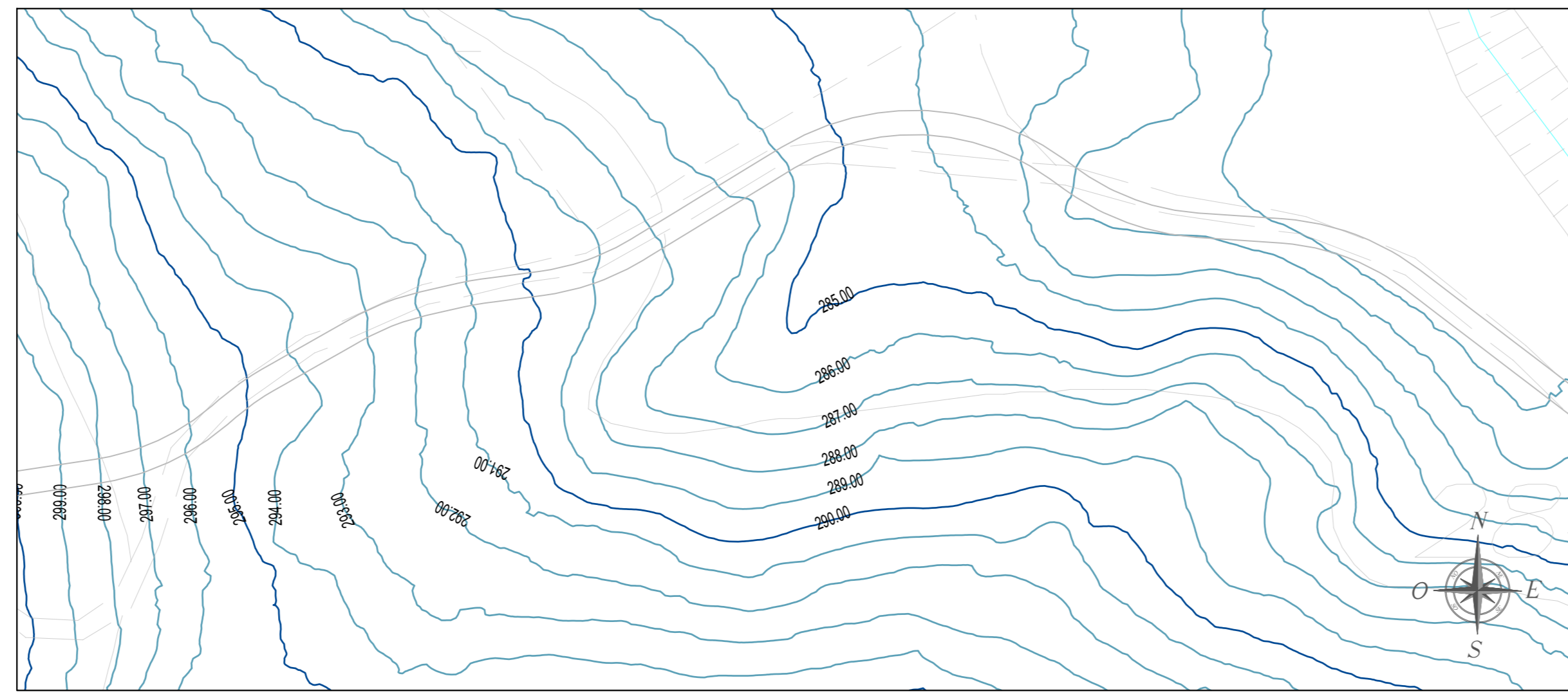
QUADRO 24 - Scala 1:1.000
