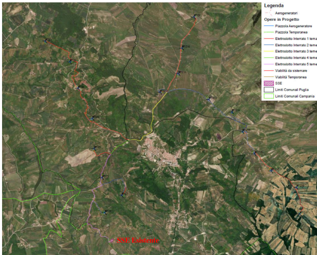
Figura 4.6. – Inquadramento su Ortofoto del nuovo Parco Eolico.
