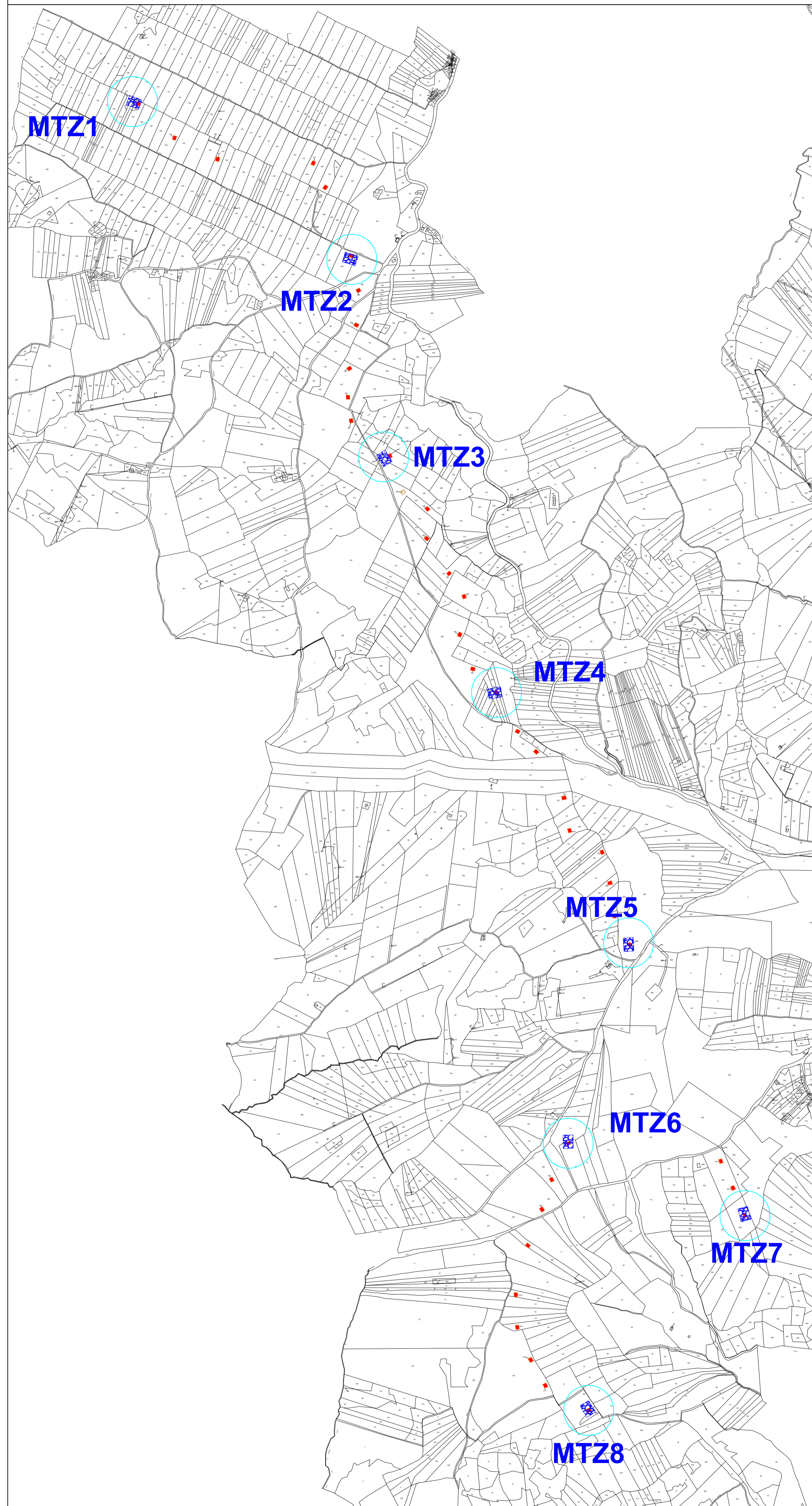
Inquadramento su base catastale Parco Eolico "MONTANZAGA" - STATO DI PROGETTO (Scala 1: 8.000)
