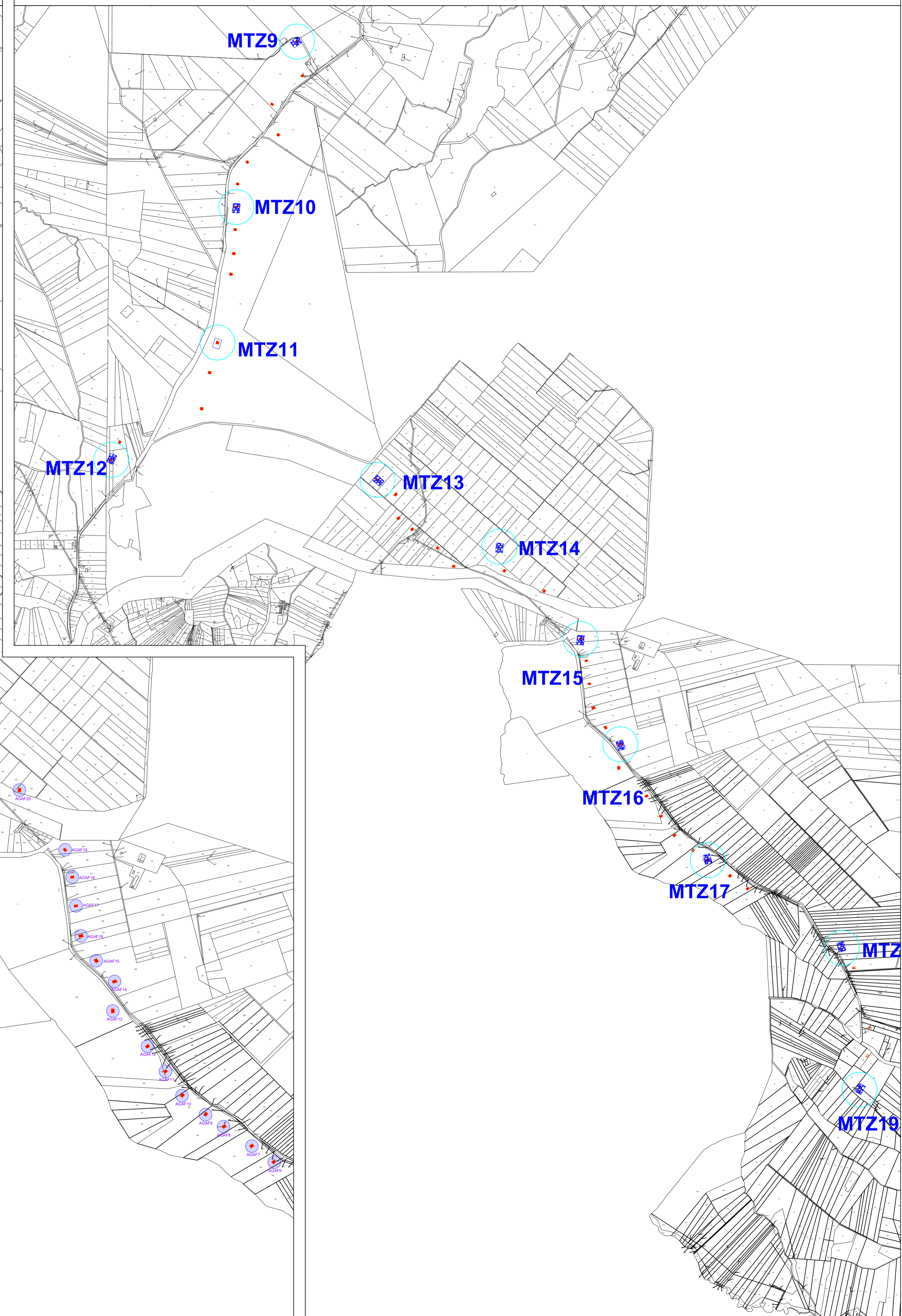
Inquadramento su base catastale aggiornato Parco Eolico "MONTANZAGA" - STATO DI PROGETTO (Scala 1: 10.000)
