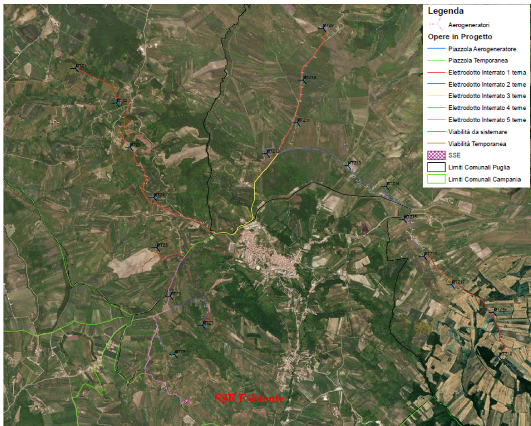
Figura 2.5. – Inquadramento su Ortofoto del futuro parco eolico.
