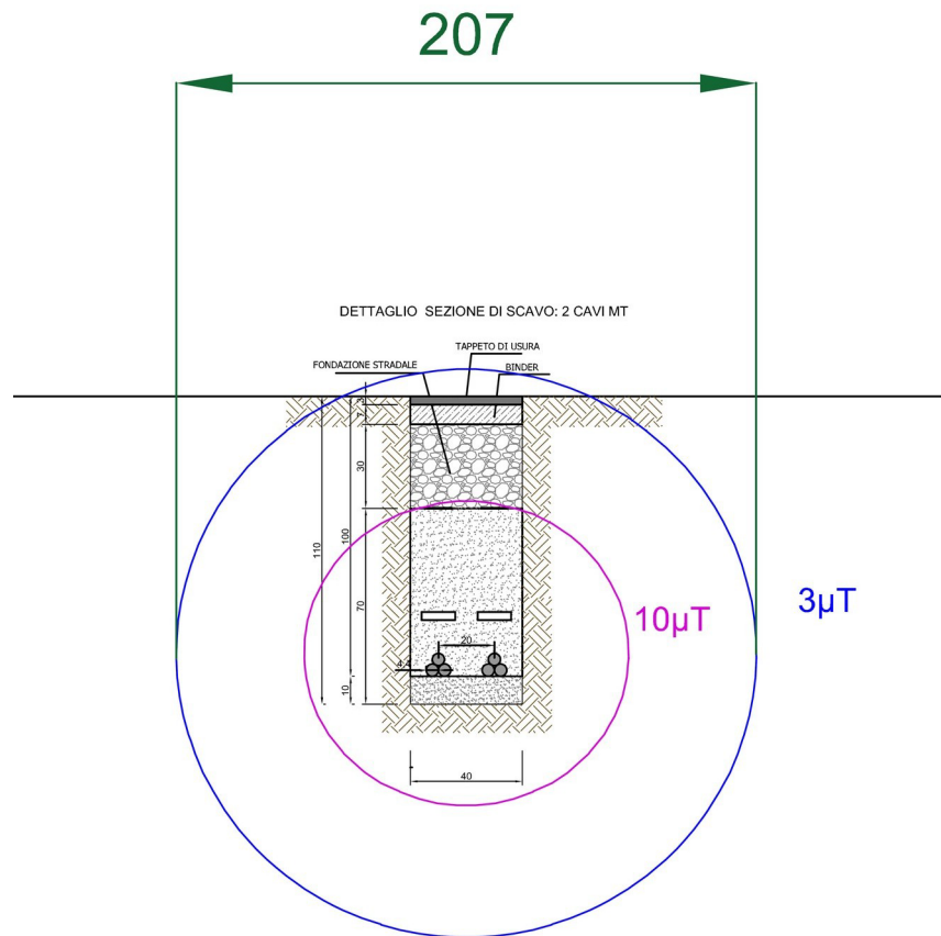
Fascia di rispetto cavidotto 30 kV
