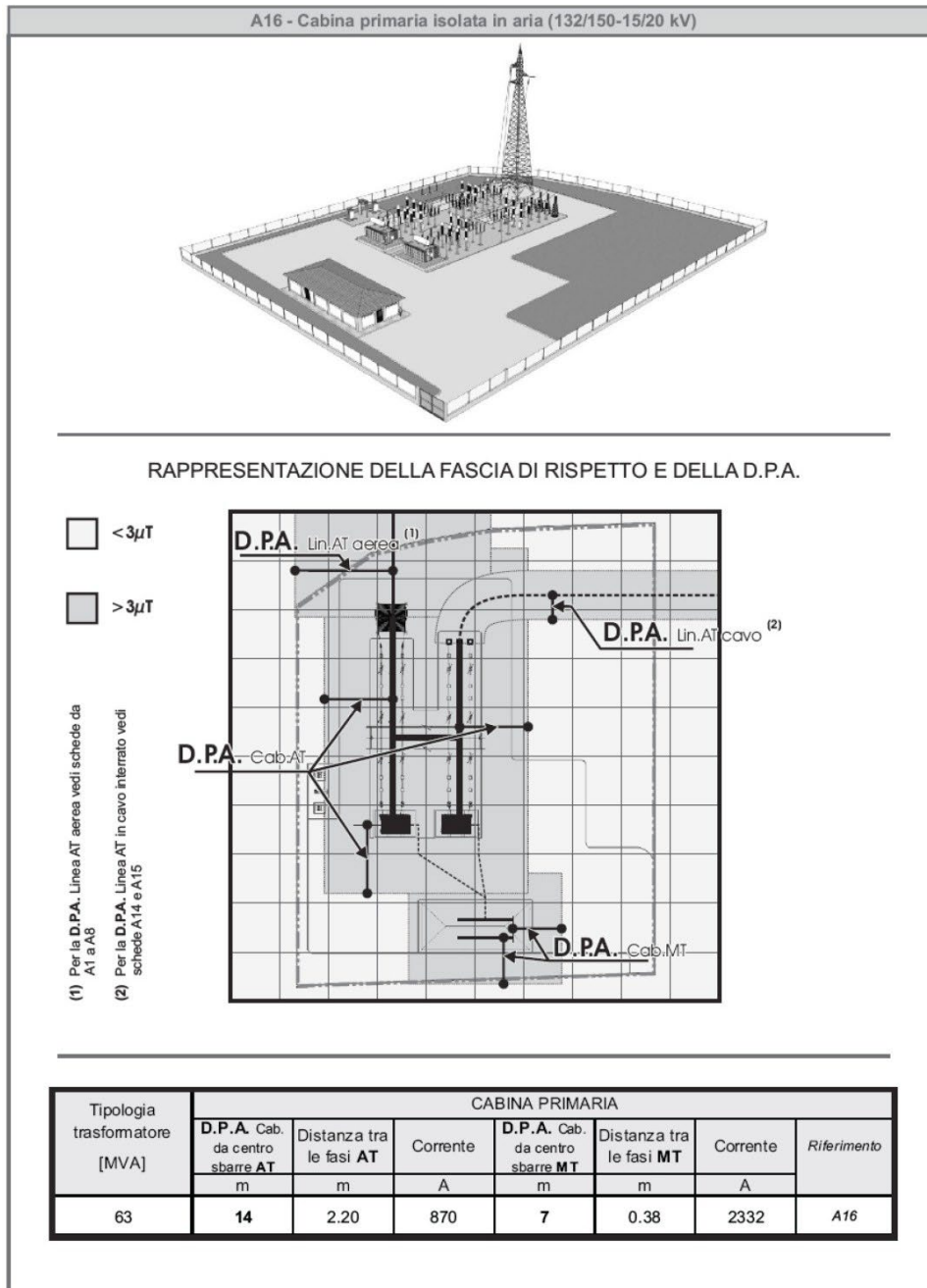
Scheda A16 e -distribuzione: fascia di rispetto cabina primaria 150 kV
