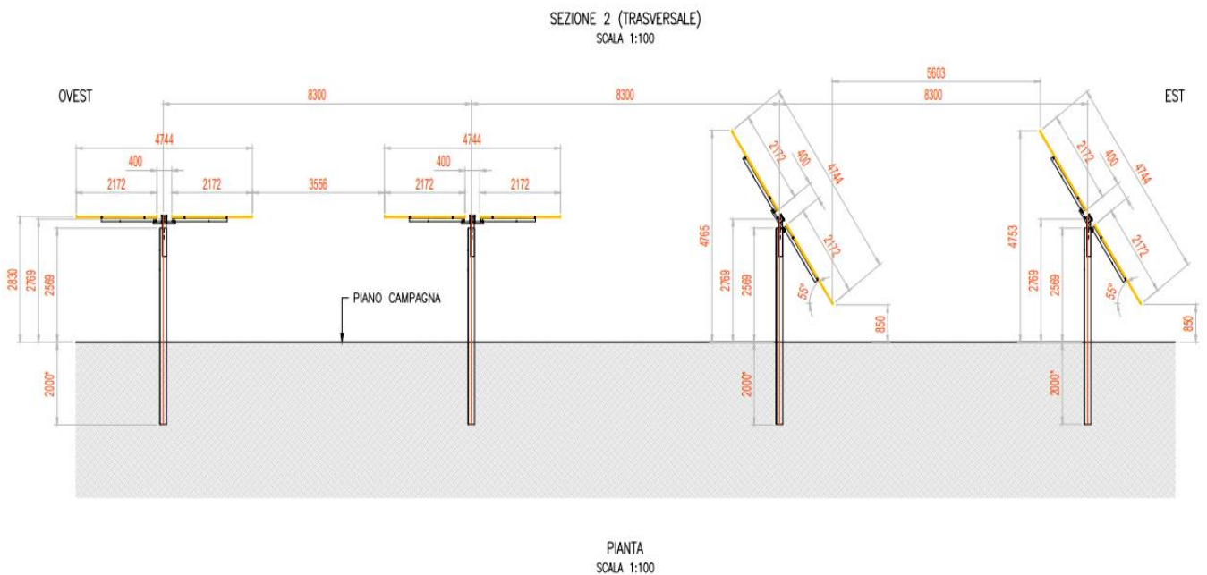
Particolare strutture sostegno moduli pannelli e distanze di campo (interfila m 8.3)
