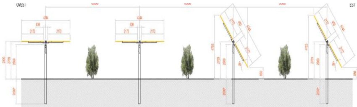
Profilo dell'interfila dell'impianto olivicolo (larghezza m. 8,3)
