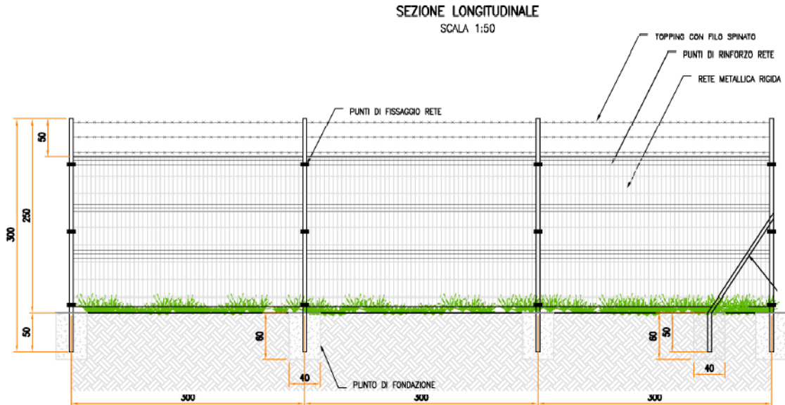
Figura 4.4: Particolare recinzione
