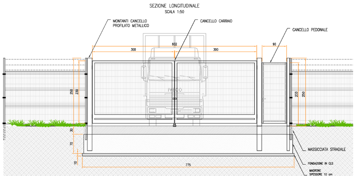
Figura 4.5: Particolare accesso
