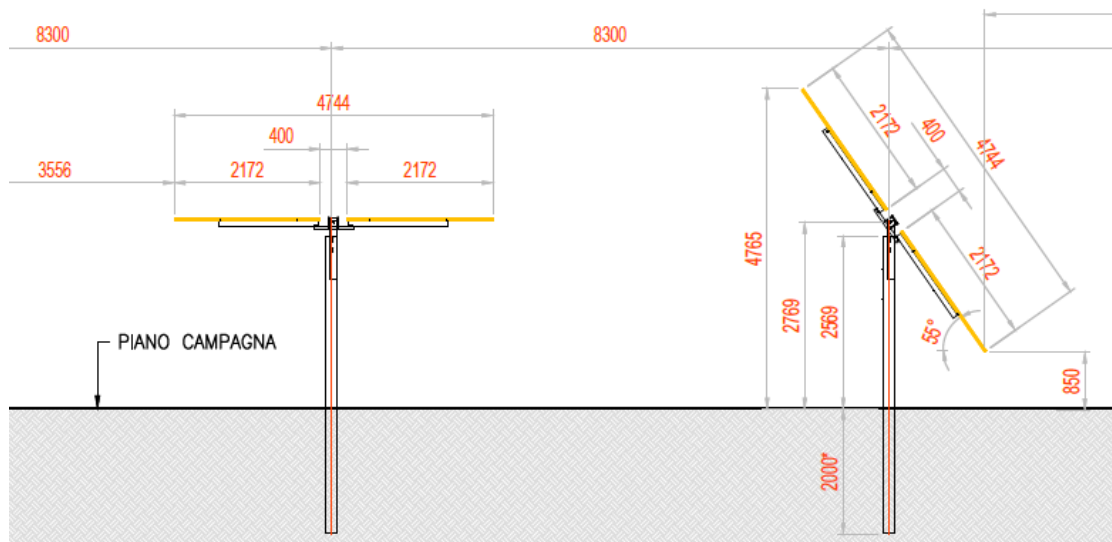
Figura 4.3: Particolare strutture di sostegno moduli
