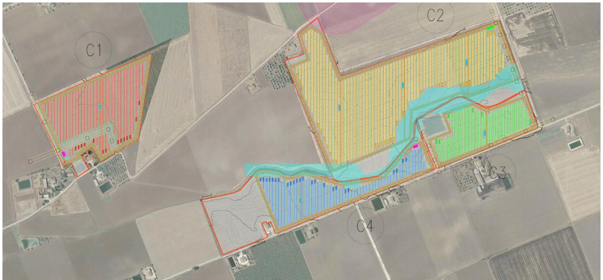
Figura 4.1: Layout di progetto – area nord
