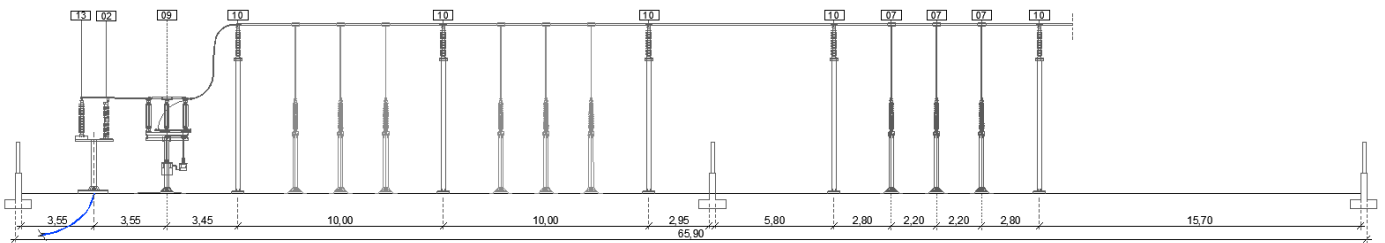
Figura 1 – Planimetria Elettromeccanica
