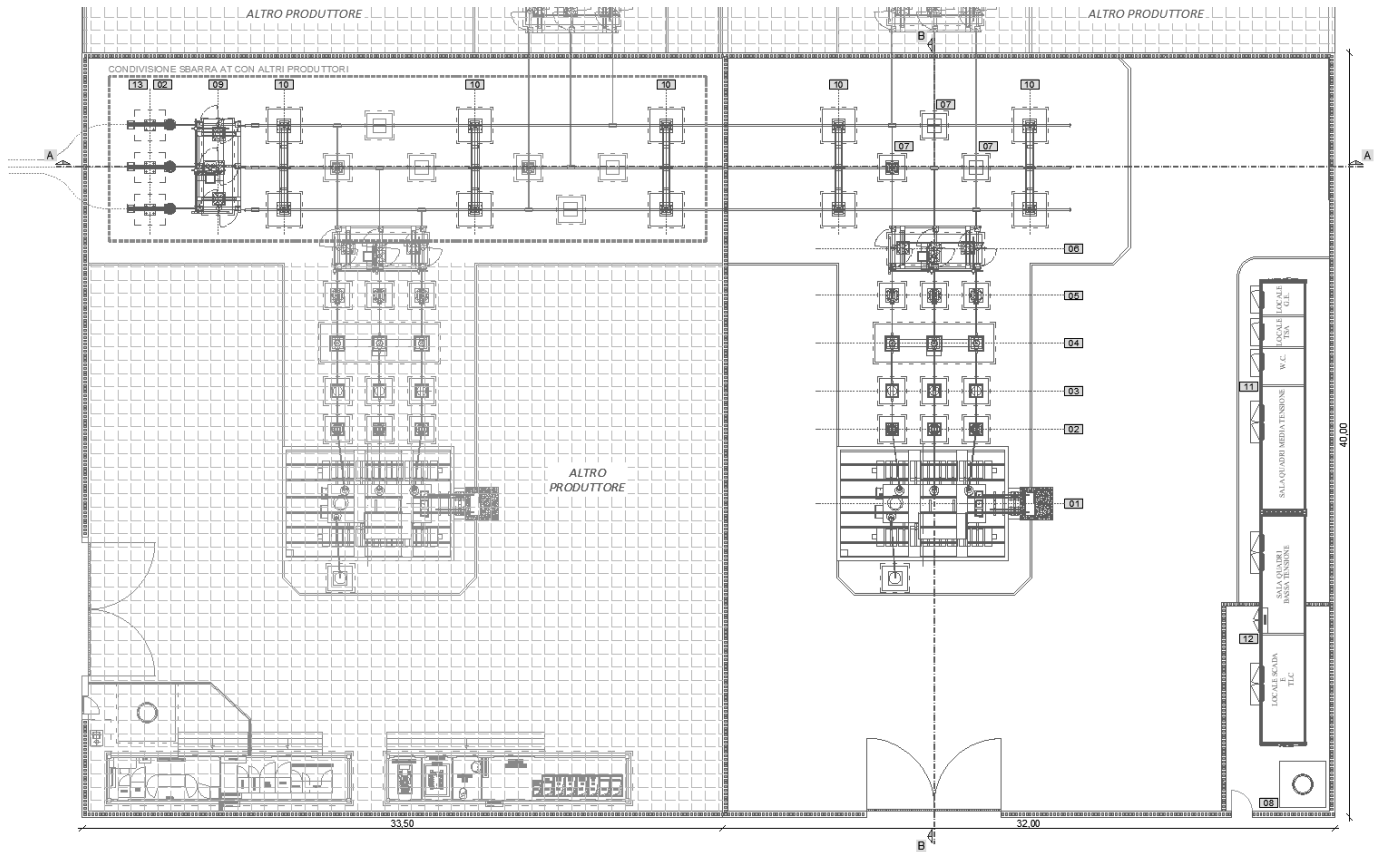
Figura 1 – Planimetria Elettromeccanica
