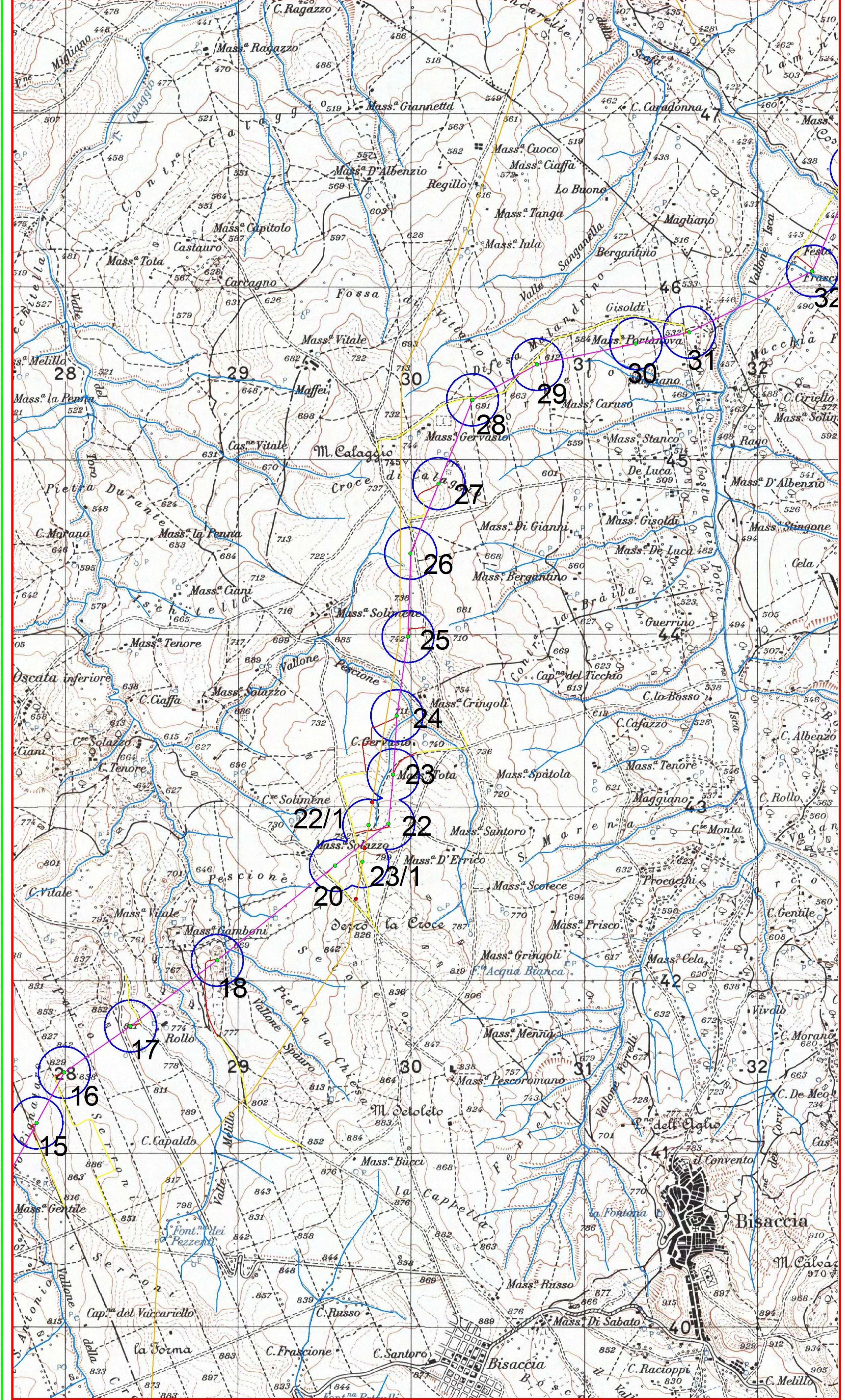
Rappresentazione dei trallici del riquadro n°2 dell'elettrodotto aereo con i rispettivi buffer di 150 m e reticoli IGM - scal 1:10000
