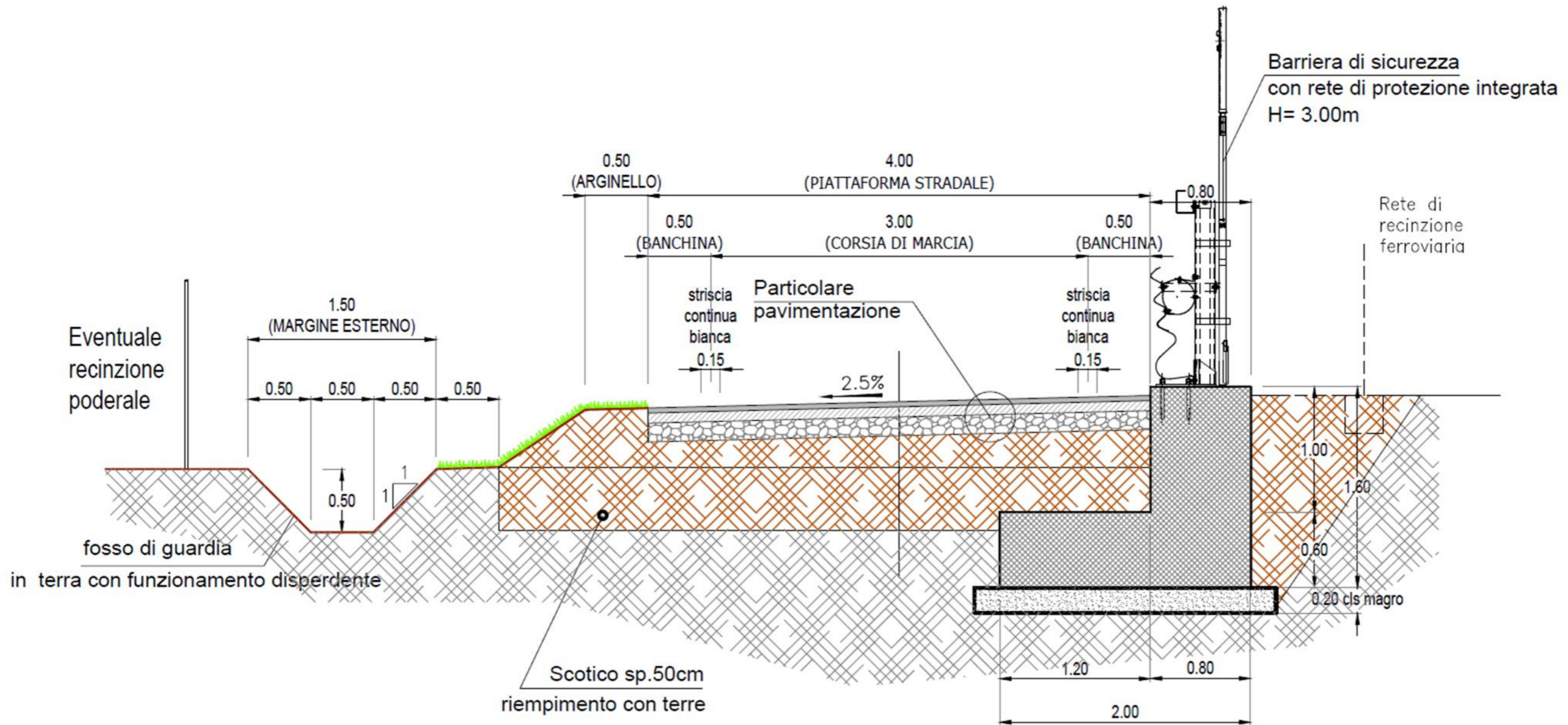
Figura 6.4 – Sezione tipo: configurazione a tetto con barriere di sicurezza
