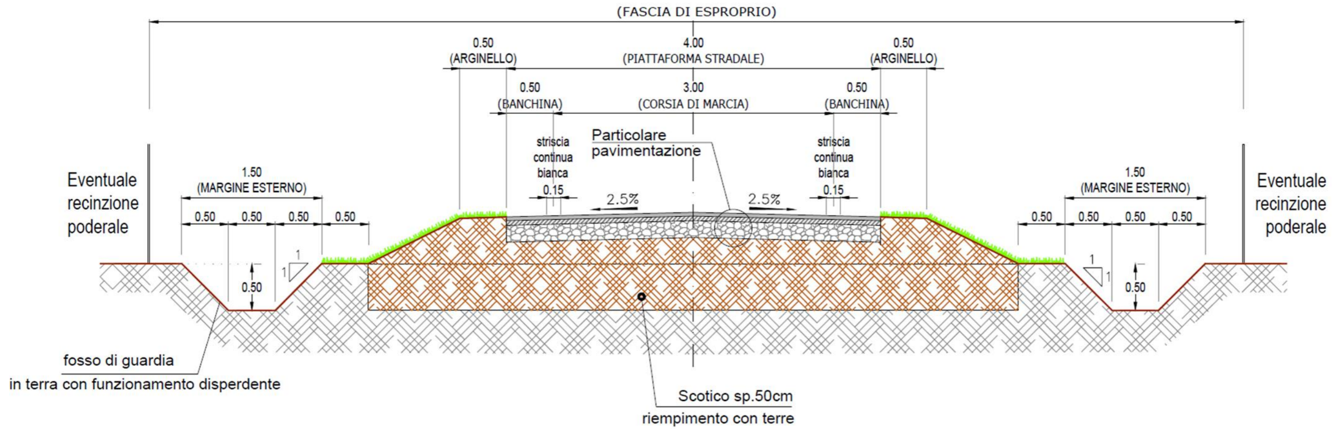
Figura 6.5 – Sezione tipo ricuciture: configurazione a schiena
