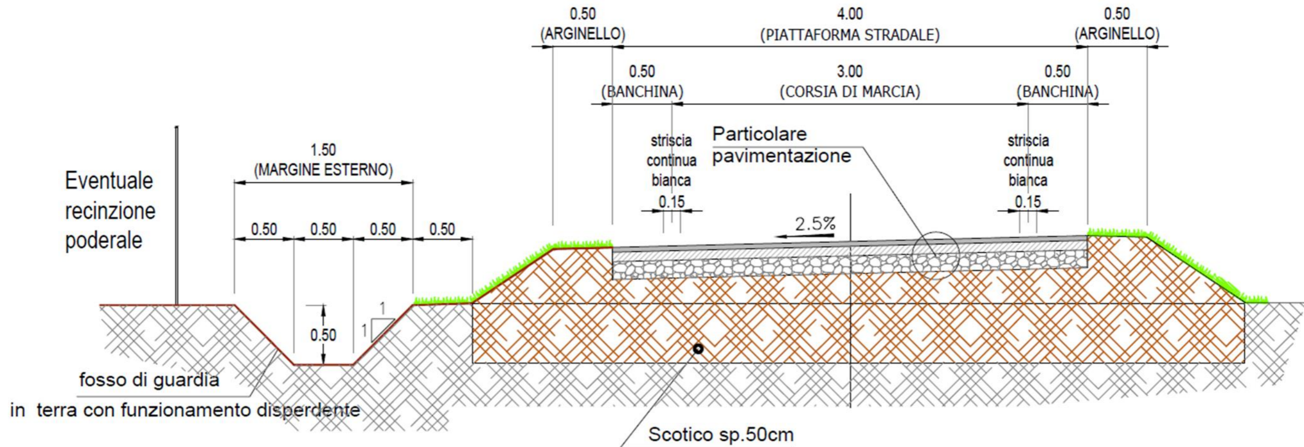
Figura 6.3 – Sezione tipo ricuciture: configurazione a tetto
