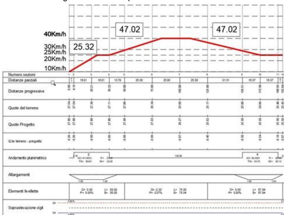
Diagramma velocità planimetrica – Ricucitura n.12
