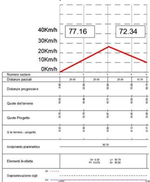
Diagramma velocità planimetrica – Ricucitura n.18
