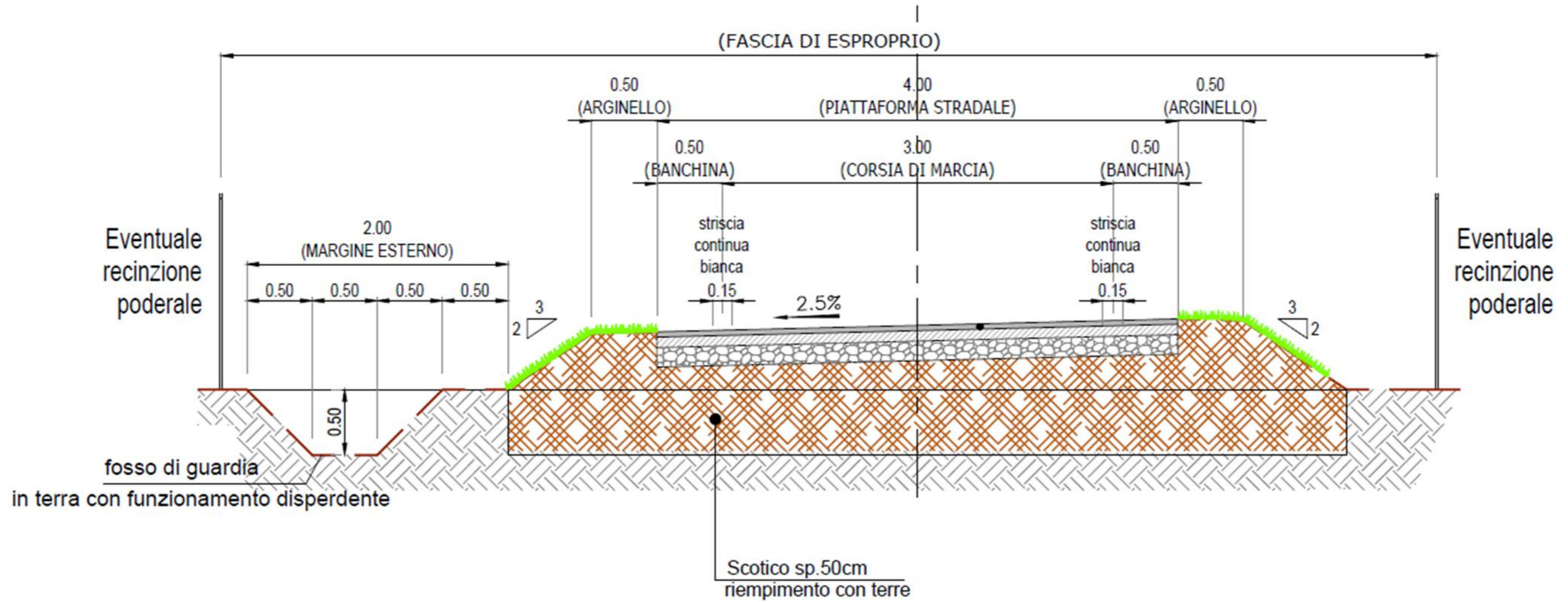
Figura 6.2 – Sezione tipo ricuciture: configurazione a tetto
