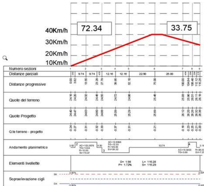
Diagramma velocità planimetrica – Ricucitura n.14
