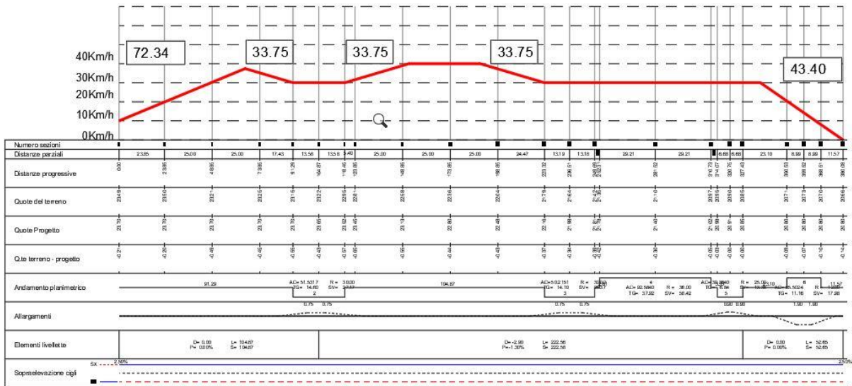
Diagramma velocità planimetrica – Ricucitura n.13
