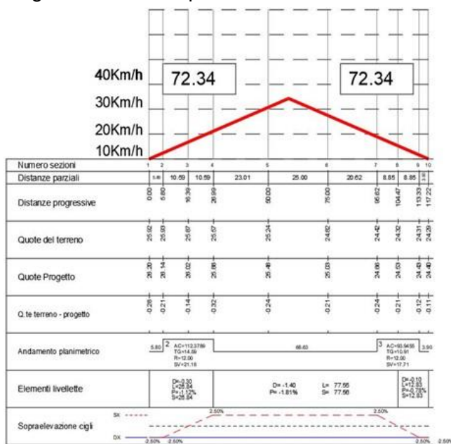
Diagramma velocità planimetrica – Ricucitura n.15
