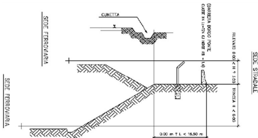
Figura 11.1 – Posizionamento della barriera
