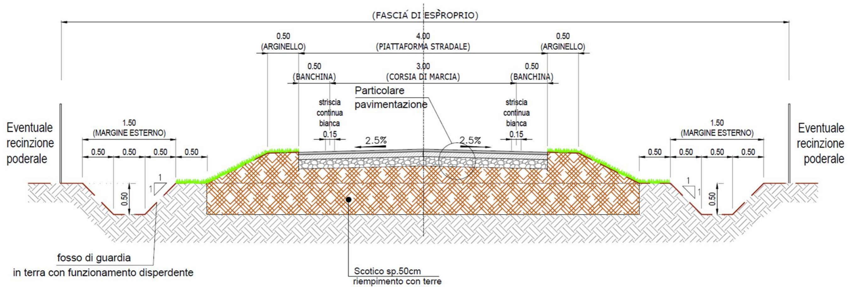
Figura 6.4 – Sezione tipo ricuciture: configurazione a schiena
