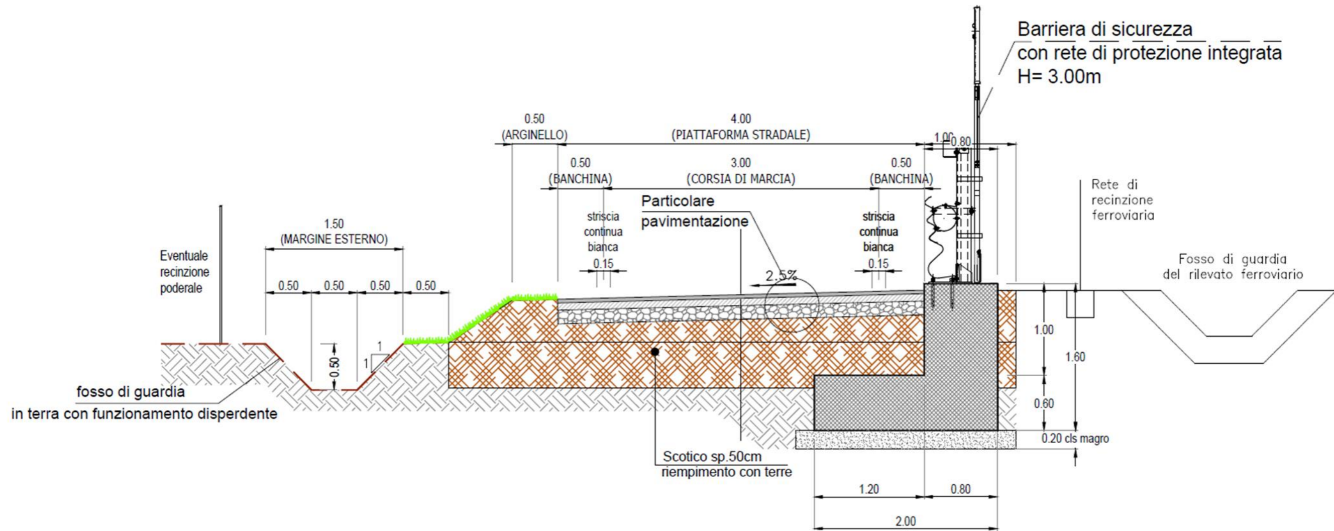
Figura 6.3 – Sezione tipo: configurazione a tetto con barriere di sicurezza
