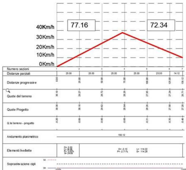
Diagramma velocità planimetrica – Ricucitura n.16
