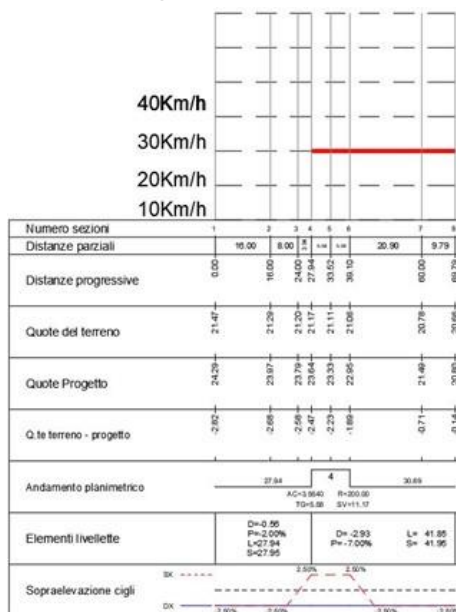
Diagramma velocità planimetrica – Ricucitura n.17bis
