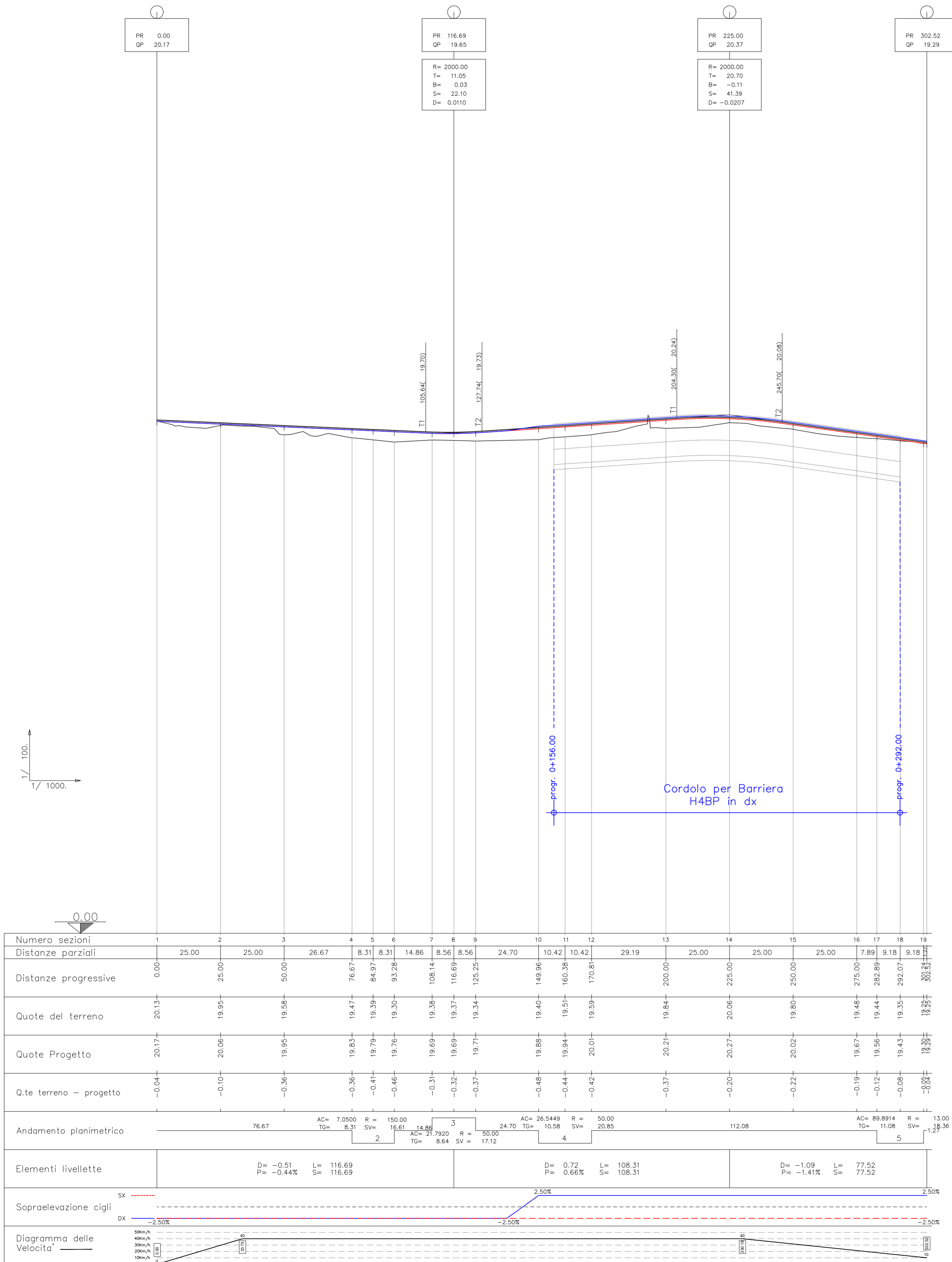
PROFILO LONGITUDINALE RICUCITURA N. 24
