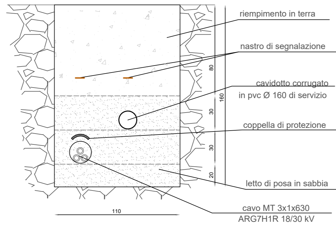
SEZIONE TIPO B - B' Scala 1:20
