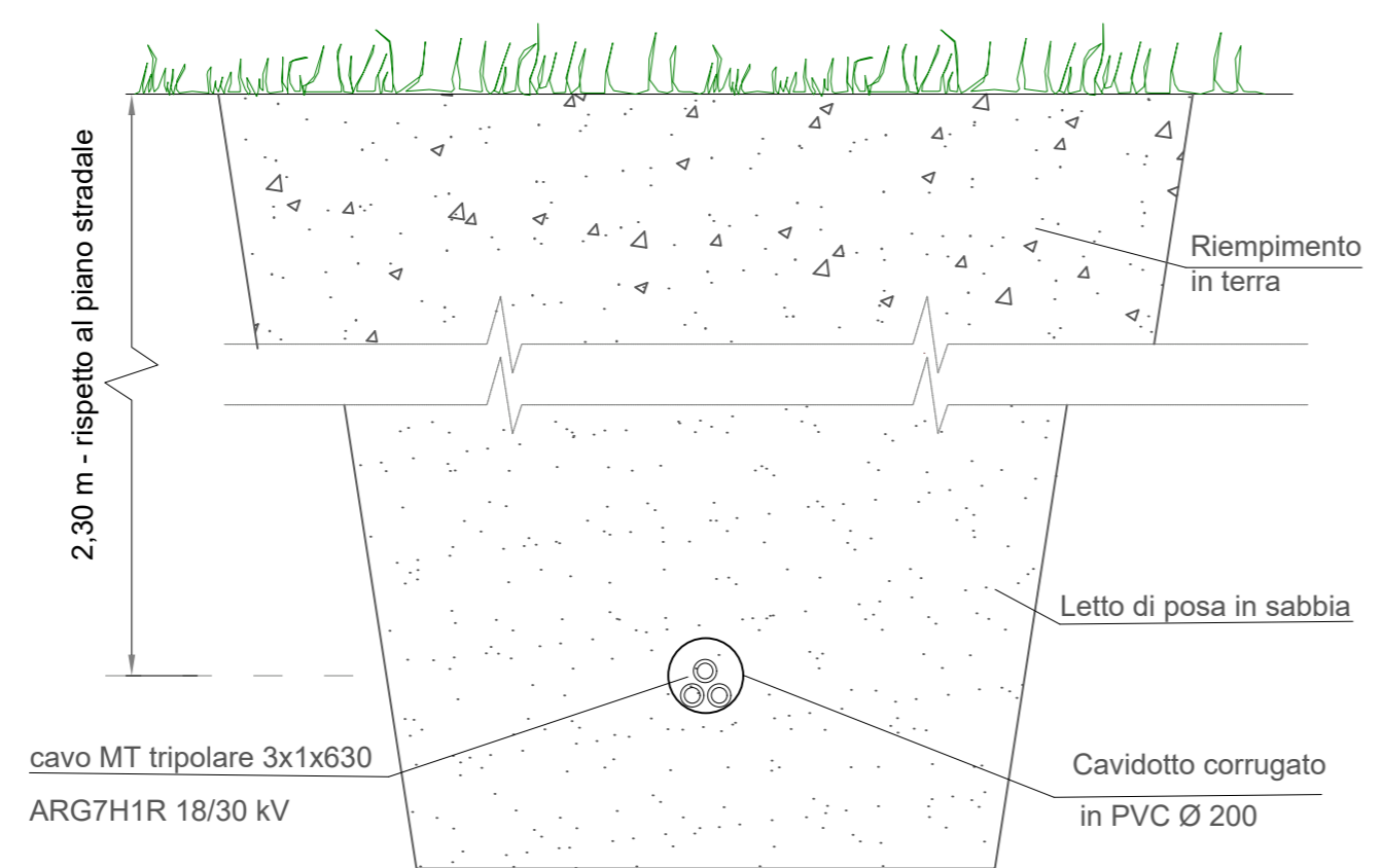
SEZIONE TIPO M - M' SEZIONE DI CAVIDOTTO IN PERFORAZIONE TELEGUIDATA A TRIFOGLIO Scala 1:20
