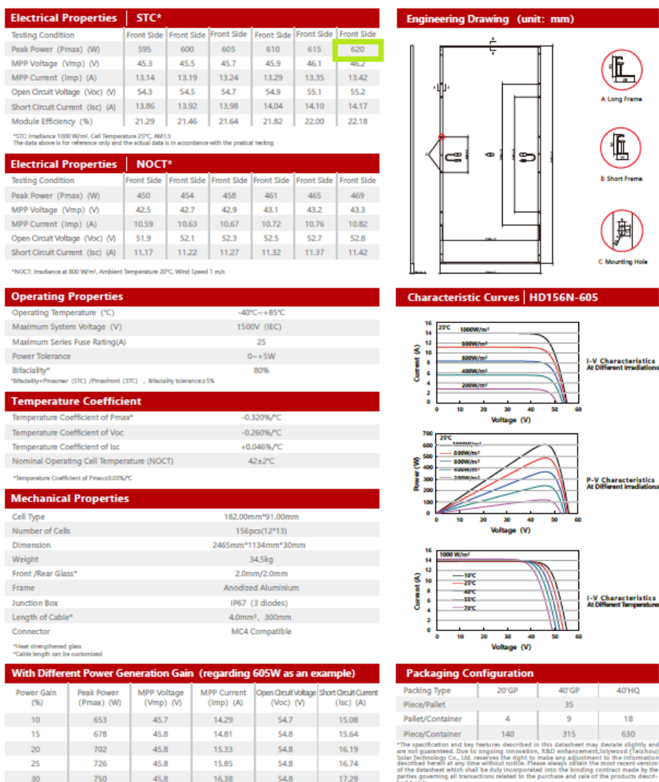
Figura 1 - Dati tecnici pannelli FV
