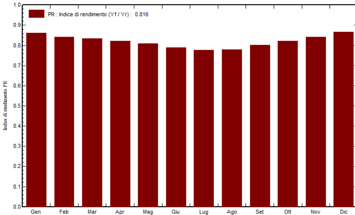
Indice di rendimento PR
