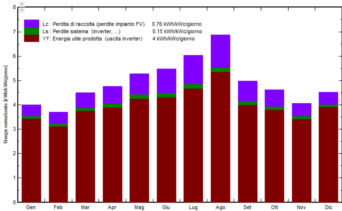
Produzione normalizzata ( per KW insatllato): Potenza nominale 19986 kWp
