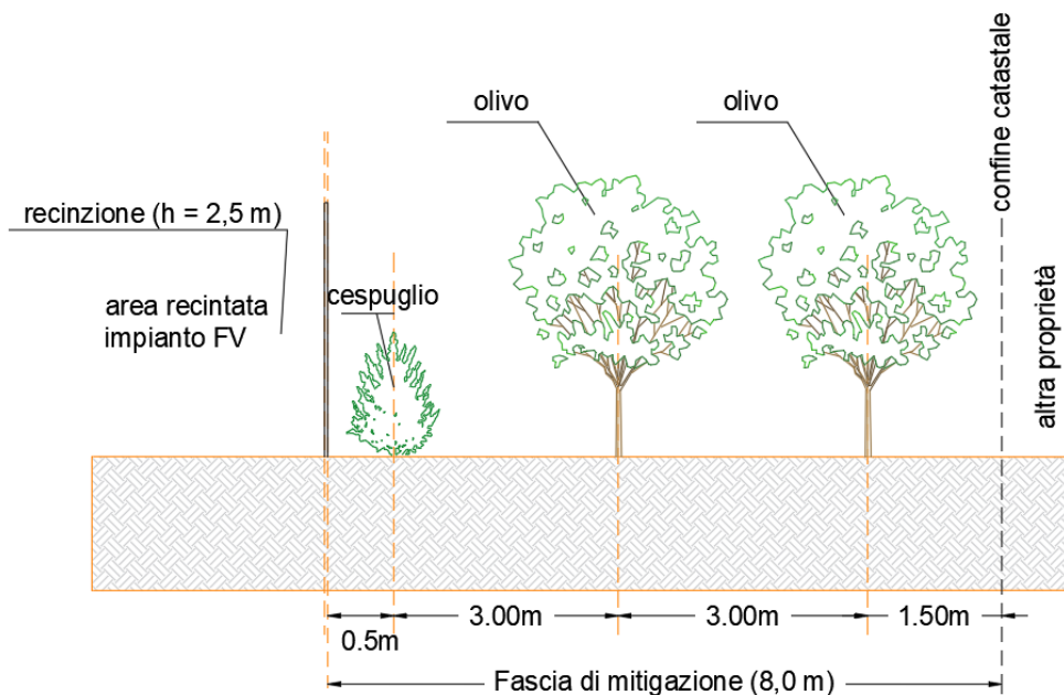
Figure 14.4. – Sezione tipo Aree coltivate.
