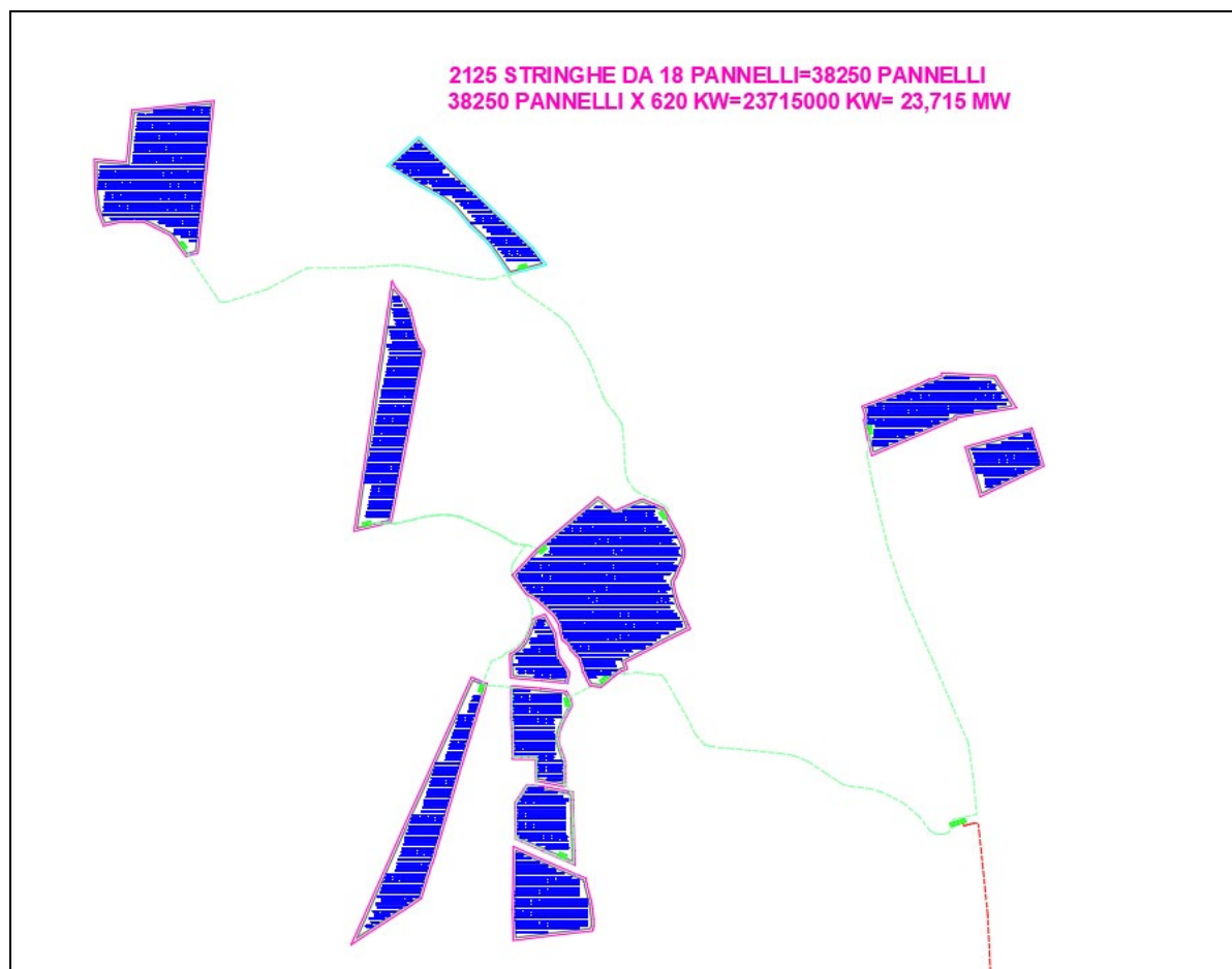
Figura 7.2 – Layout del sistema fotovoltaico con supporti fissi
