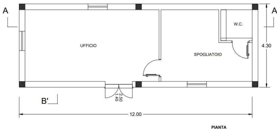
Figura 6.11. – Schematizzazione in pianta locale di servizio.
