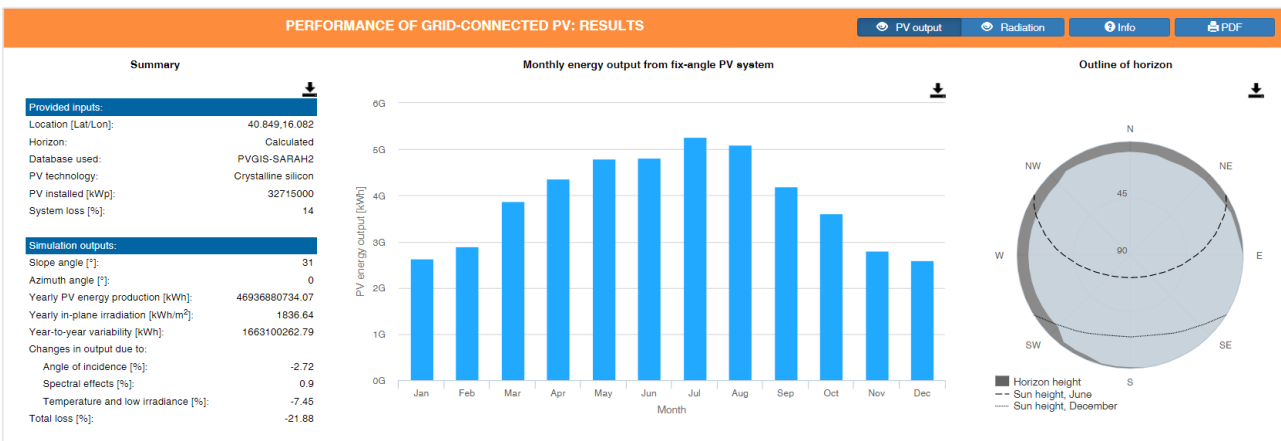
Figura 7.7 - Simulazione di produttività annua del sistema fotovoltaico con supporti fissi
