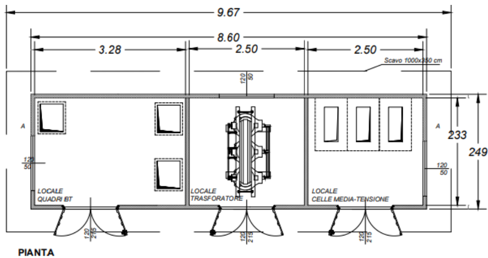
Figura 6.9. – Schematizzazione in pianta cabina di trasformazione.
