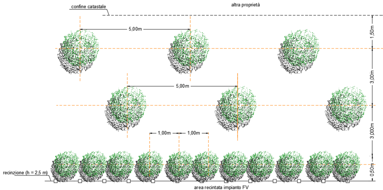
Figure 14.3. – Sezione tipo Fascia di mitigazione.
