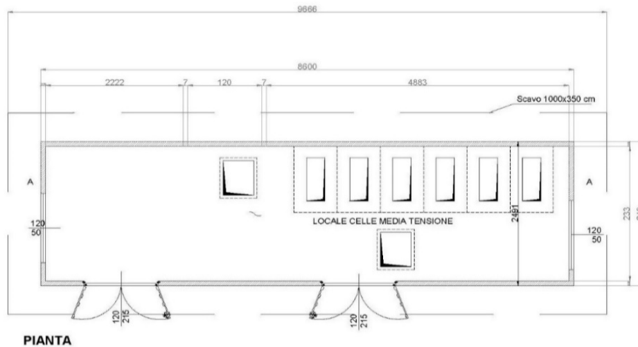
Figura 6.10. – Schematizzazione in pianta cabina di raccolta.
