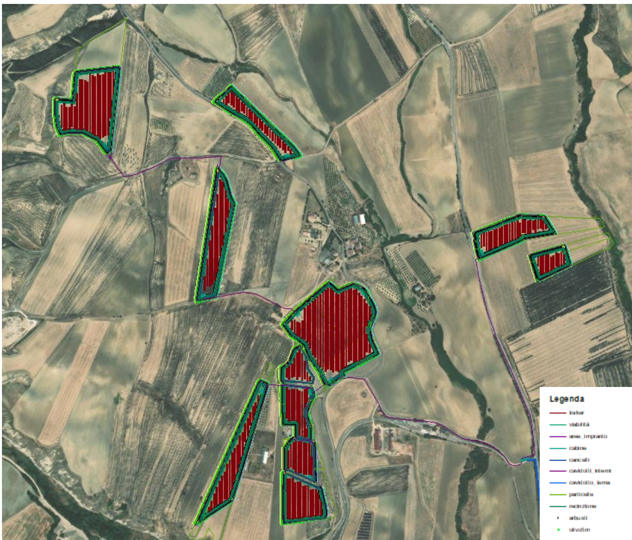
Figura 6.4. – Layout dell’impianto agrivoltaico.
