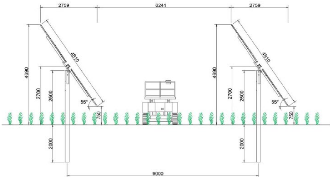
Figure 14.2. – Sezione tipo Aree coltivate
