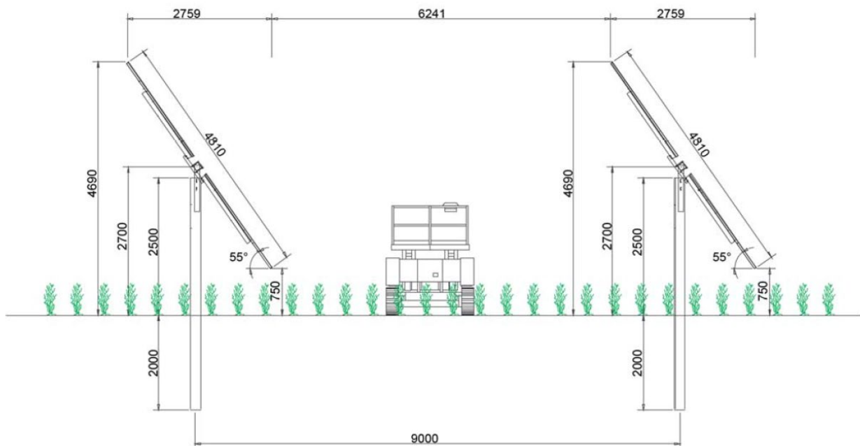
Figura 6.6. – Vista laterale dei tracker con inclinazione 0^\circ e 55^\circ .
