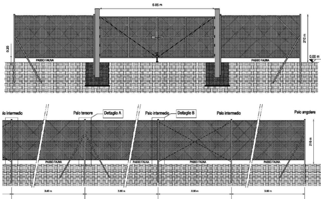
Figura 6.12. – Cannello di accesso e recinzione impianto agrivoltaico.
