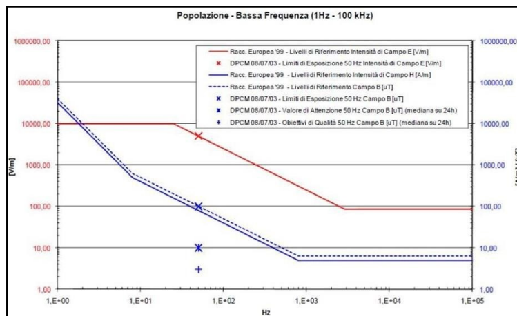
Figura 3.12. – Livelli esposizione Bassa Frequenza (1Hz – 100 kHz).
