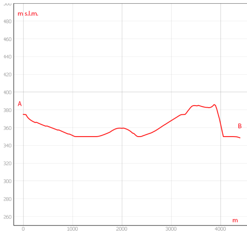
Sezione morfologica del terreno- Punto di presa n°1
