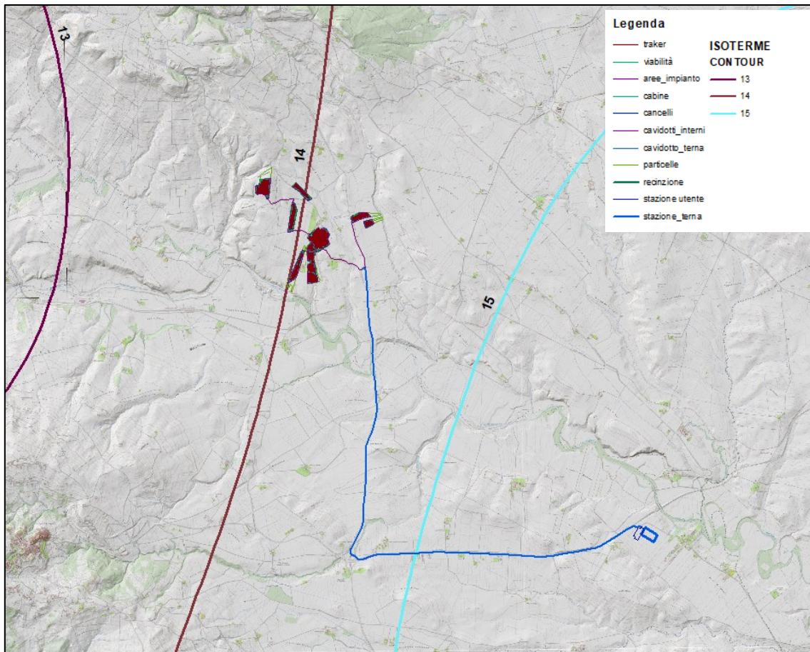
Figura 27- Mappa delle Isotherme
