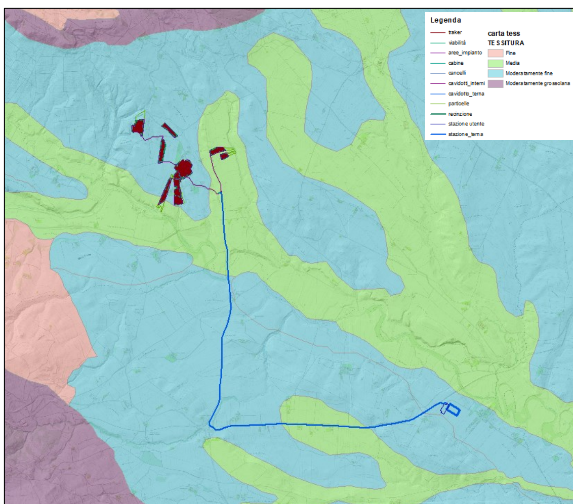
Figura 35 - Carta della tessitura dell'orizzonte superficiale
