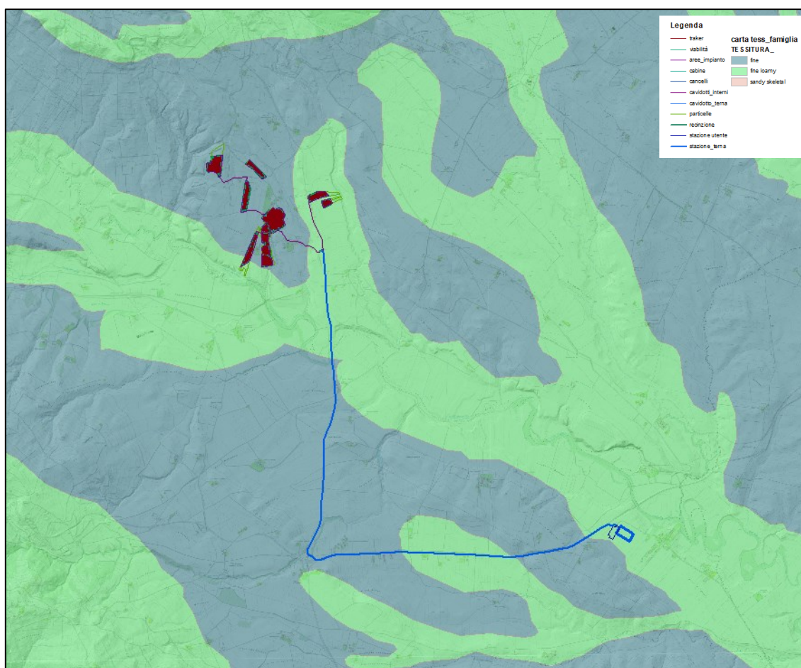
Figura 36 - Carta della tessitura areale di progetto
