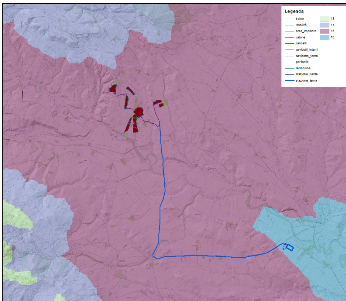
Figura 28 - Temperatura media annua areale di progetto
